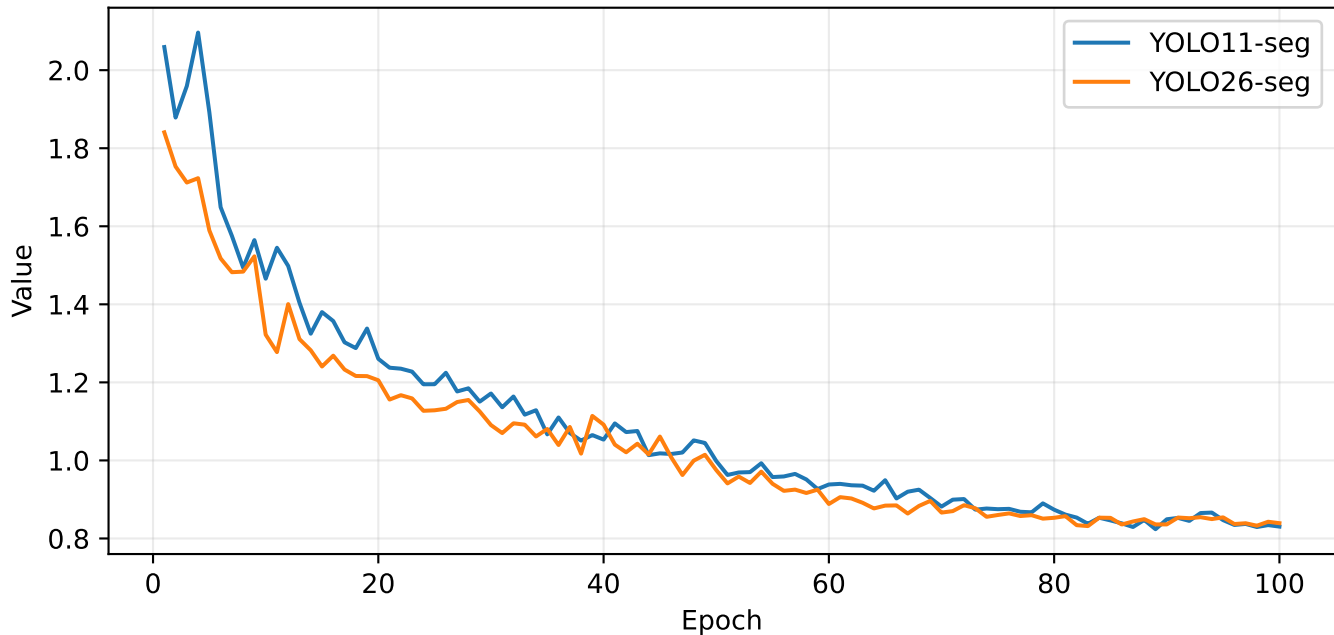
Val Seg Loss
