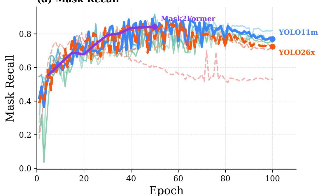
(d) Mask Recall
