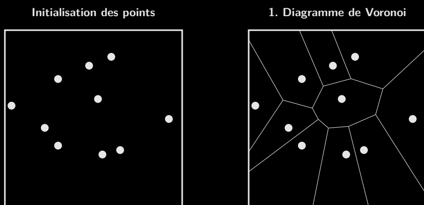
FIGURE 1 – Processus de génération du maillage dual de Voronoi à partir d'un nuage de points.
