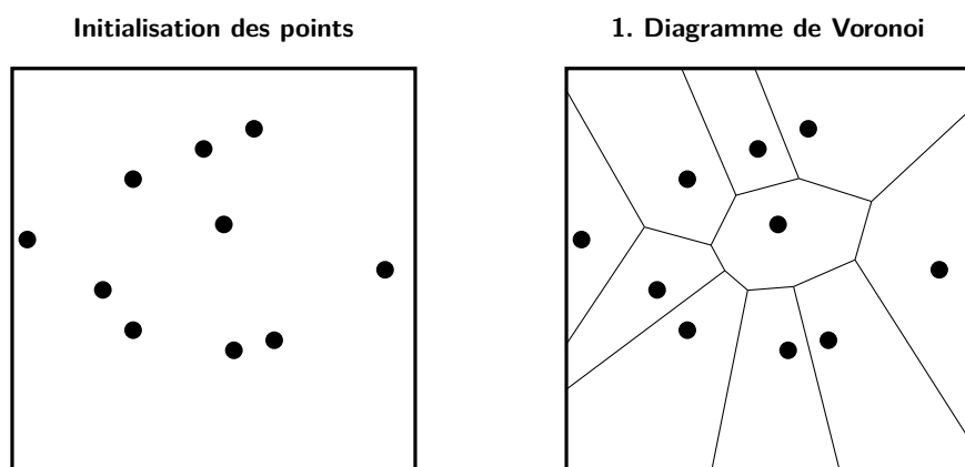
FIGURE 1 – Processus de génération du maillage dual de Voronoi à partir d'un nuage de points.
