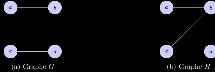
FIGURE 1 – Illustration des graphes G et H
