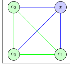
FIGURE 2 – Graphe G avec un 3-cycle C et un 3-sommet x
