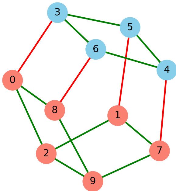
Heuristic partition
