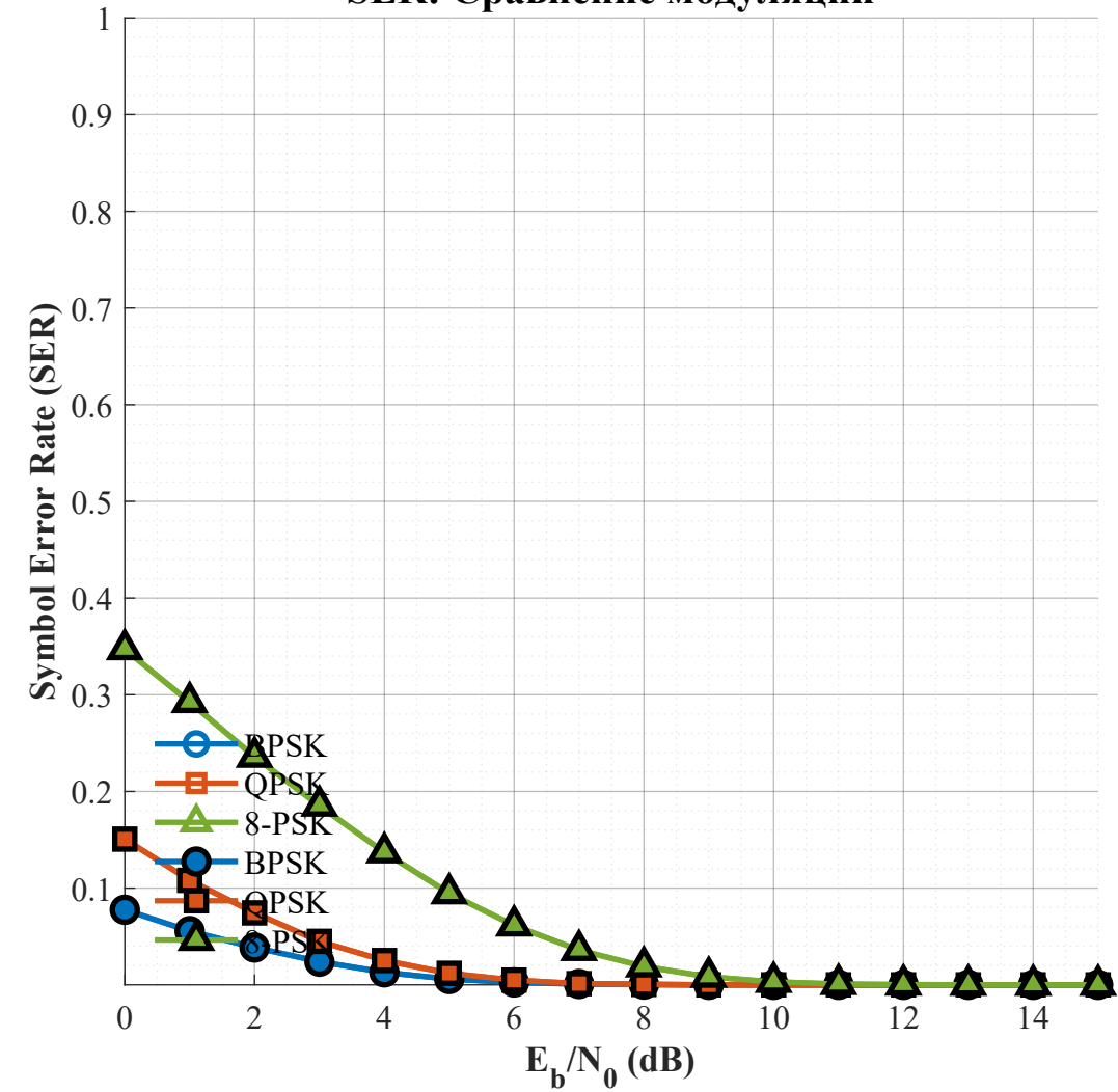
SER: Сравнение модуляций
