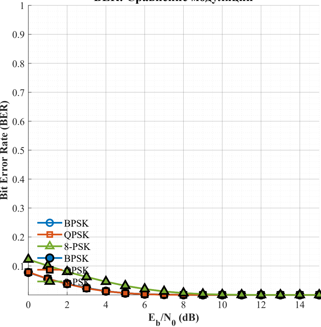
BER: Сравнение модуляций
