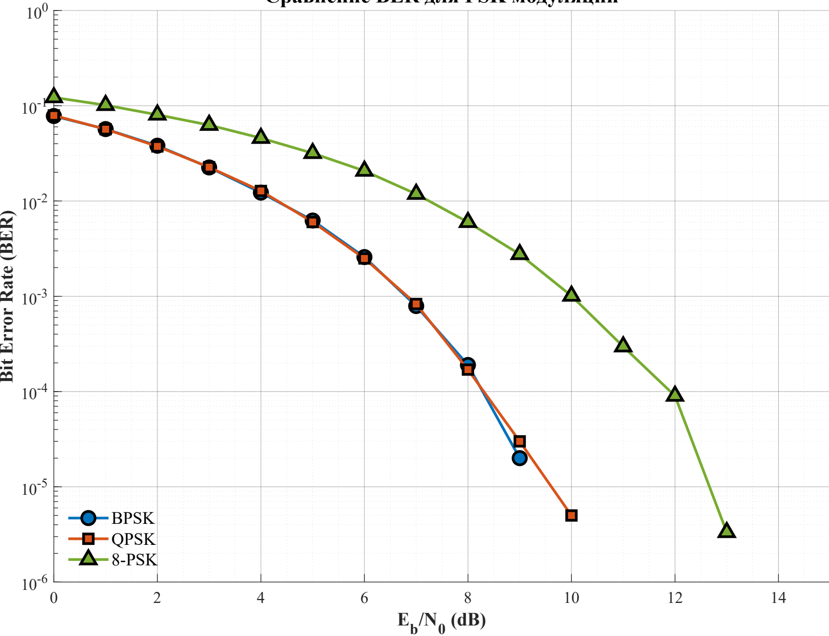
Сравнение BER для PSK модуляций
