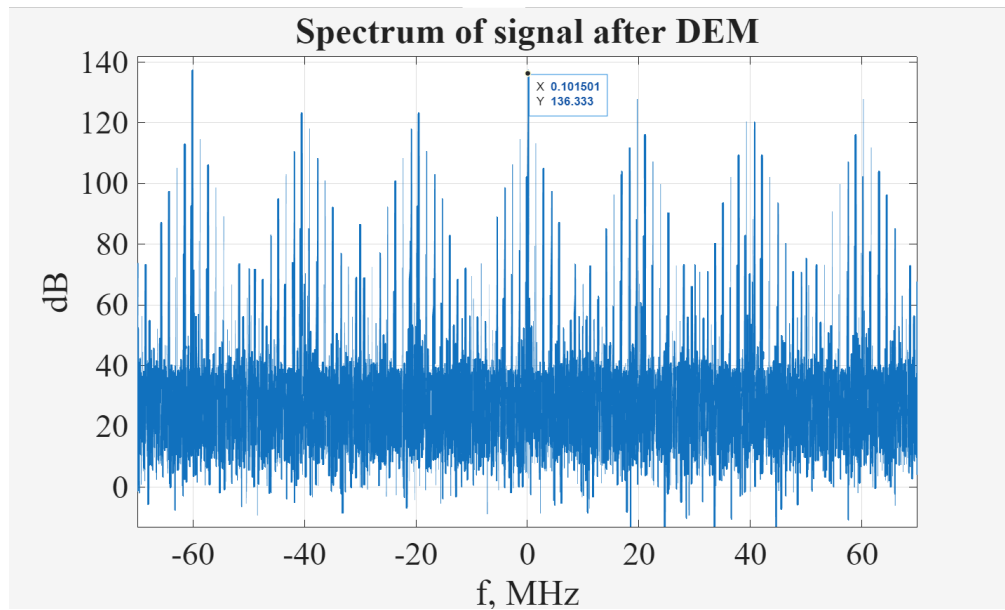
Рис. 9 — Спектр сигнала на выходе DEM
