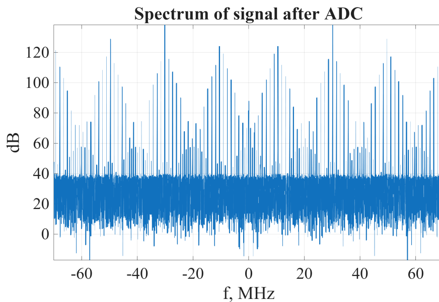
Рис. 5 — Спектр после АЦП
