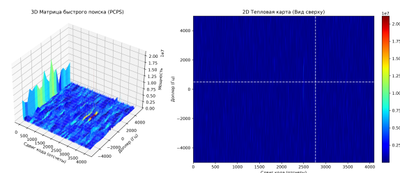
Рис. 3 — Двумерная функция неопределенности, полученная на выходе детектора мощности power_detector : 3D-профиль (слева) и проекция на плоскость «задержка – Доплер» (справа)
