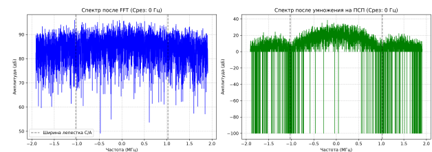
Рис. 2 — Спектральная плотность мощности сигнала на промежуточных каскадах: на выходе прямого БПФ (слева) и после перемножения со спектром опорной ПСП (справа)
