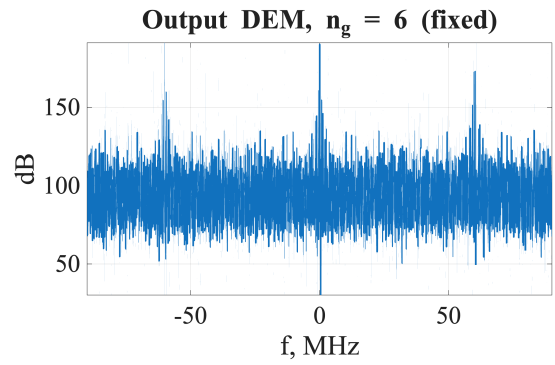
Рис. 10 — Спектр на выходе DEM ( n_g = 6 )
