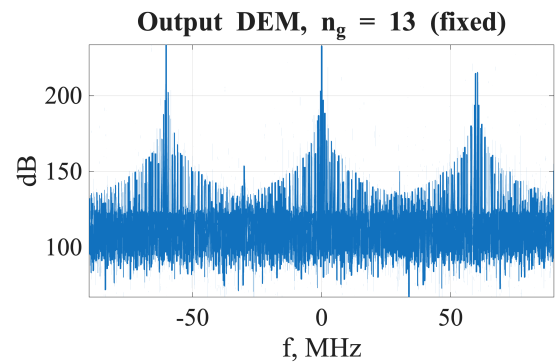
Рис. 13 — Спектр на выходе DEM ( n_g = 13 )
