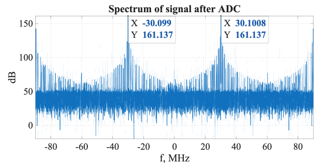
Рис. 5 — Спектр сигнала после АЦП
