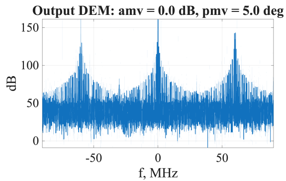
Рис. 17 — Фазовый разбаланс ( 5^\circ )
