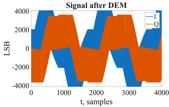
Рис. 8 — Квадратуры на выходе DEM
