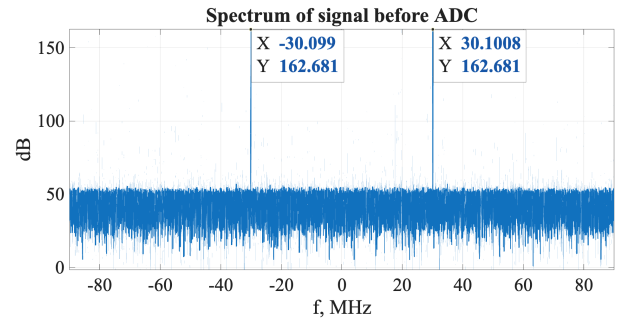
Рис. 3 — Спектр входного сигнала
