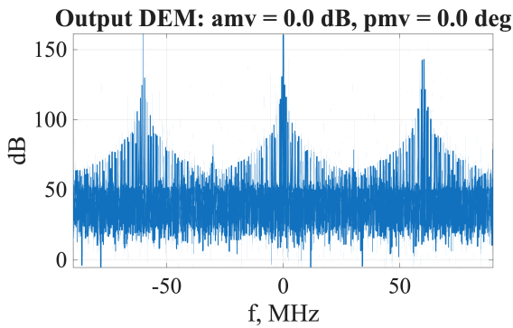
Рис. 15 — Идеальные квадратуры
