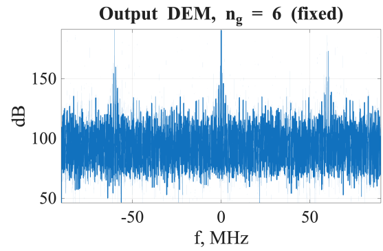
Рис. 11 — Спектр на выходе DEM ( n_g = 6 )
