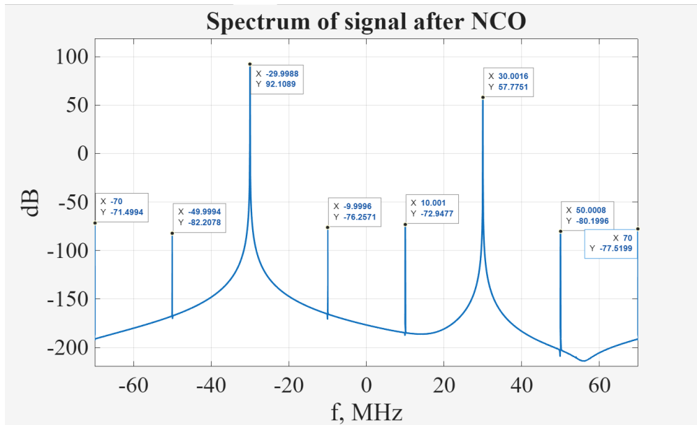
Рис. 7 — Спектр Цифрового Гетеродина
