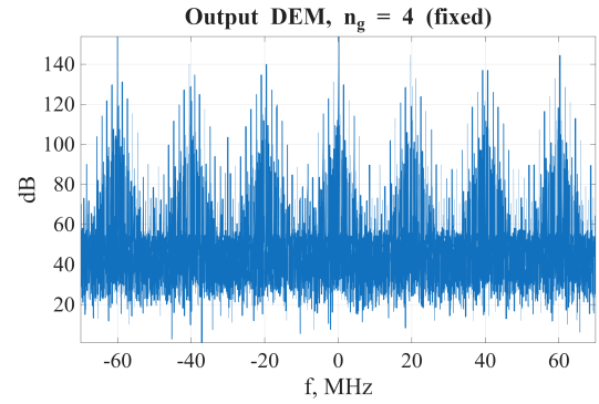
Рис. 11 — Спектр на выходе DEM ( n_g = 4 )
