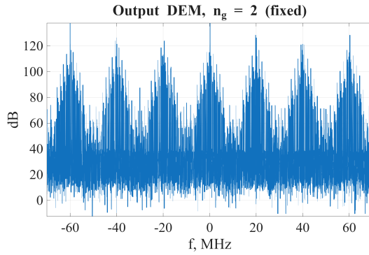
Рис. 10 — Спектр на выходе DEM ( n_g = 2 )
