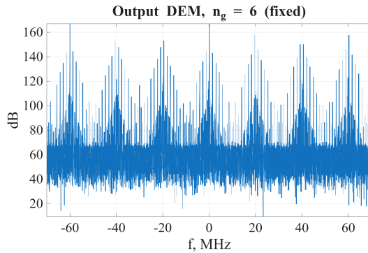
Рис. 12 — Спектр на выходе DEM ( n_g = 6 )
