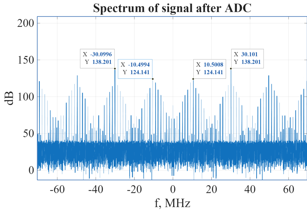
Рис. 5 — Спектр после АЦП
