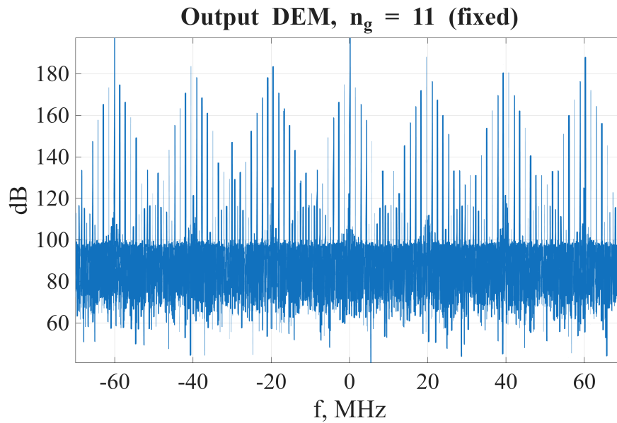
Рис. 14 — Спектр на выходе DEM ( n_g = 11 )
