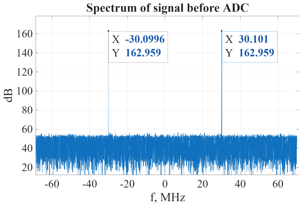
Рис. 3 — Спектр входного сигнала
