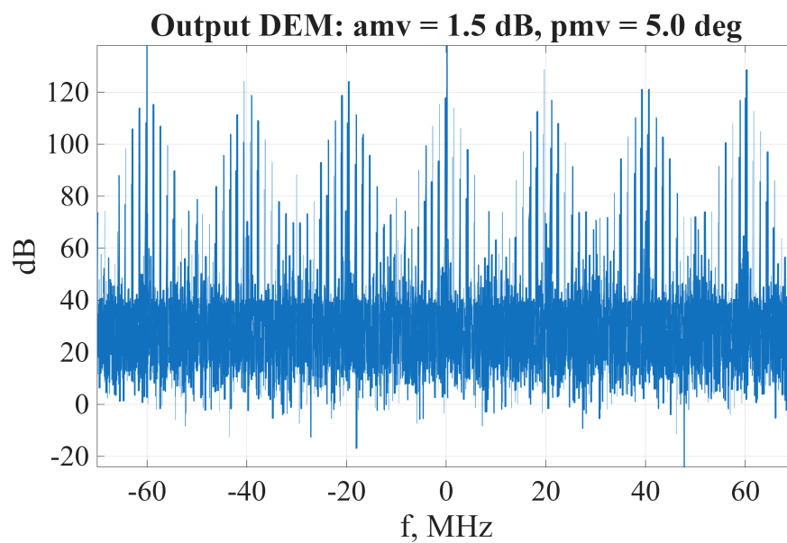
Рис. 18 — Рассогласование по амплитуде и фазе
