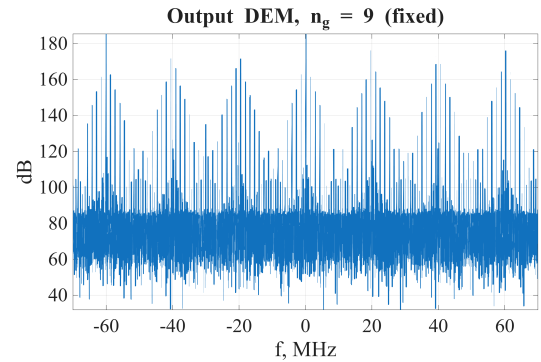
Рис. 13 — Спектр на выходе DEM ( n_g = 9 )
