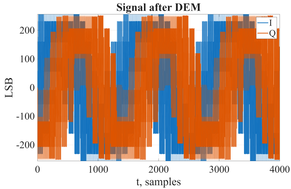
Рис. 8 — Осциллограмма каналов IQ в DEM
