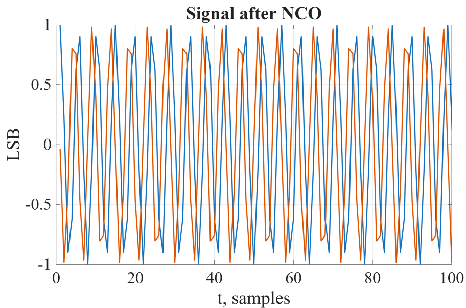
Рис. 6 — Сигнал Цифрового Гетеродина
