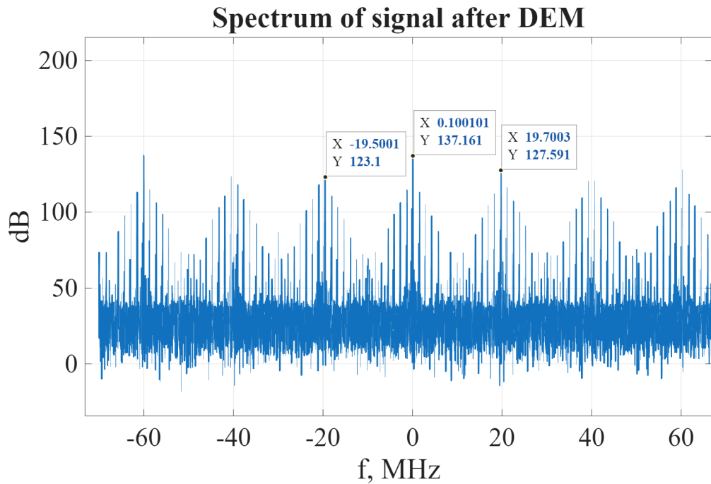
Рис. 9 — Спектр сигнала на выходе DEM
