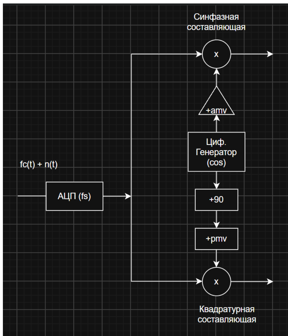
Рис. 1 — Структурная схема работы кода
