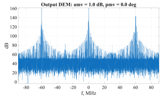
Рис. 16 — Амплитудный разбаланс (1 дБ)
