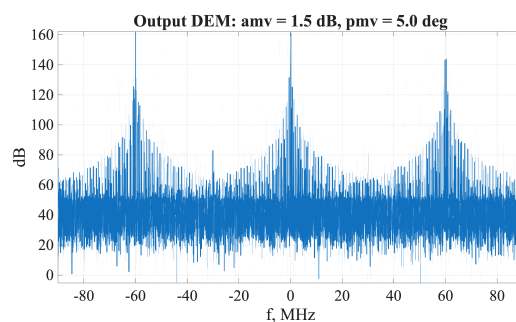
Рис. 18 — Разбаланс (1,5 дБ, 5^\circ )
