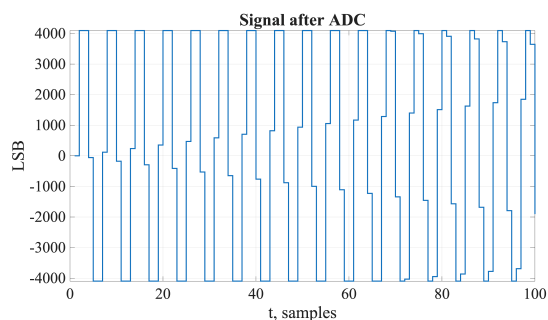
Рис. 4 — Сигнал после АЦП
