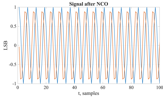
Рис. 6 — Сигнал на выходе ЦГ
