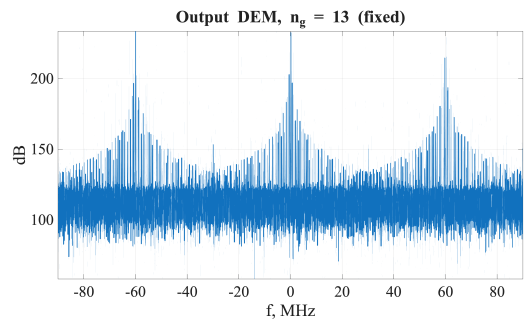
Рис. 13 — Спектр на выходе DEM ( n_g = 13 )
