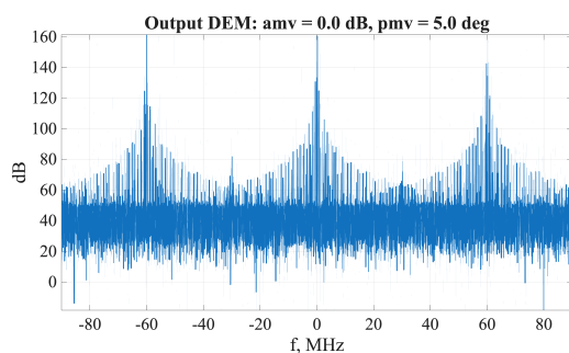
Рис. 17 — Фазовый разбаланс ( 5^\circ )
