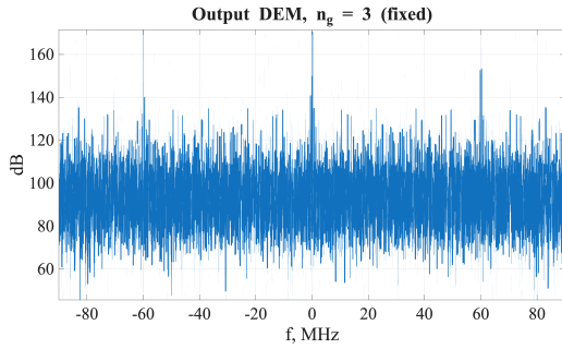
Рис. 10 — Спектр на выходе DEM ( n_g = 3 )
