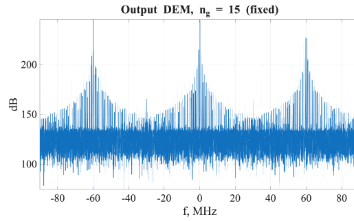
Рис. 14 — Спектр на выходе DEM ( n_g = 15 )
