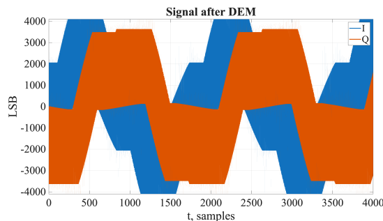
Рис. 8 — Квадратуры на выходе DEM
