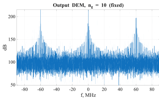
Рис. 12 — Спектр на выходе DEM ( n_g = 10 )
