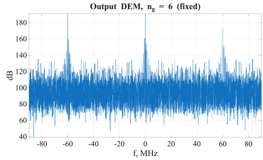
Рис. 11 — Спектр на выходе DEM ( n_g = 6 )
