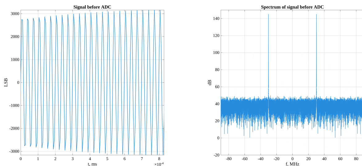
а) Осциллограмма
