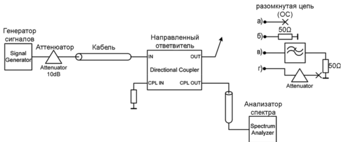
Рис. 3 — Структурная схема измерения модуля коэффициента отражения [118;1:3ис помощью направленного ответвителя
