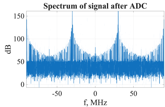
Рис. 4 — Спектр сигнала после АЦП
