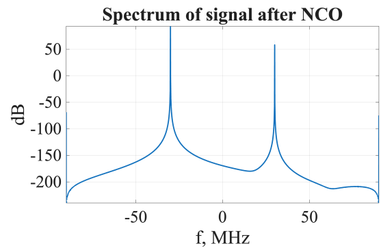
Рис. 6 — Спектр сигнала ЦГ
