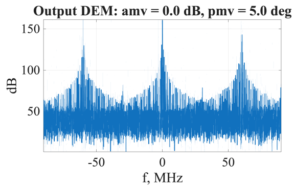
Рис. 16 — Фазовый разбаланс ( 5^\circ )
