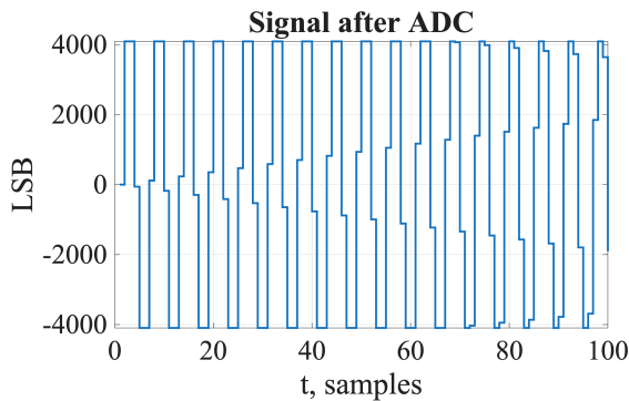
Рис. 3 — Сигнал после АЦП
