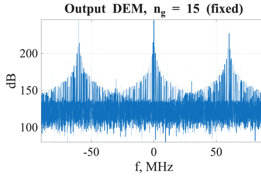
Рис. 13 — Спектр на выходе DEM ( n_g = 15 )
