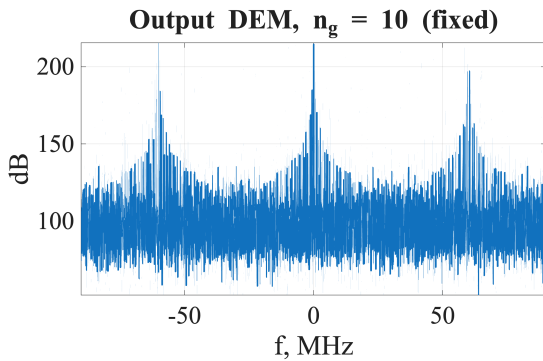
Рис. 11 — Спектр на выходе DEM ( n_g = 10 )
