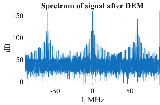
Рис. 8 — Спектр на выходе DEM
