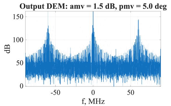
Рис. 17 — Разбаланс (1,5 дБ, 5^\circ )
