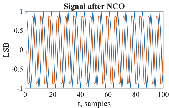
Рис. 5 — Сигнал на выходе ЦГ
