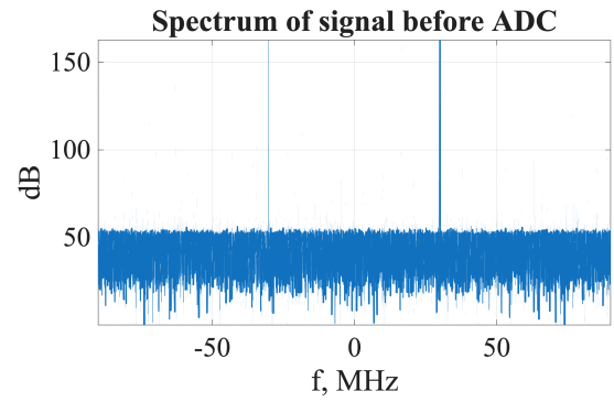
Рис. 2 — Спектр входного сигнала
