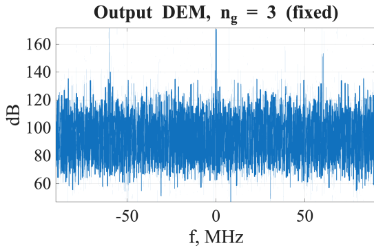
Рис. 9 — Спектр на выходе DEM ( n_g = 3 )
