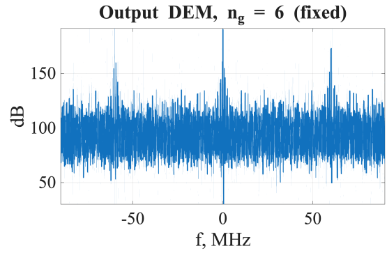
Рис. 10 — Спектр на выходе DEM ( n_g = 6 )
