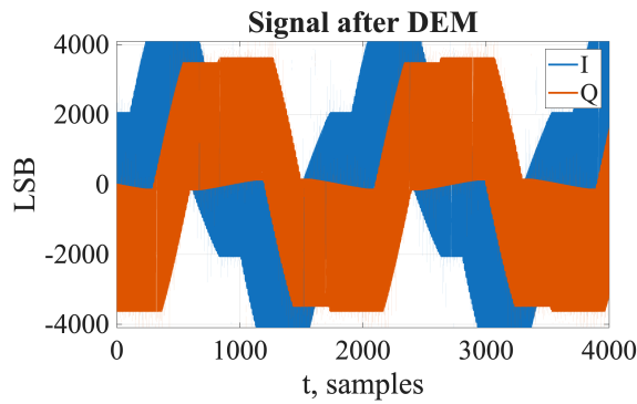
Рис. 7 — Квадратуры на выходе DEM
