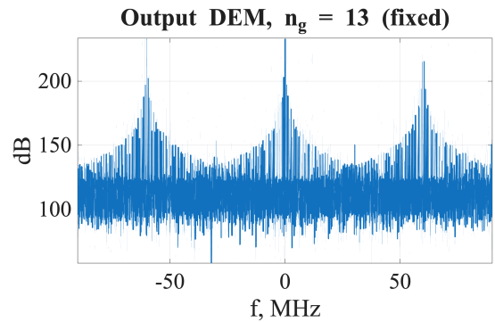
Рис. 12 — Спектр на выходе DEM ( n_g = 13 )
