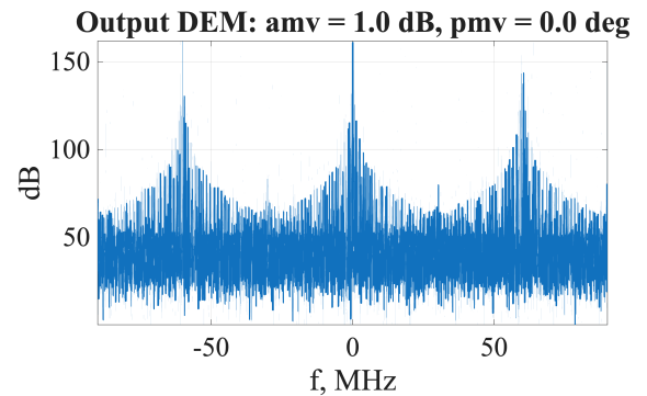
Рис. 15 — Амплитудный разбаланс (1 дБ)
