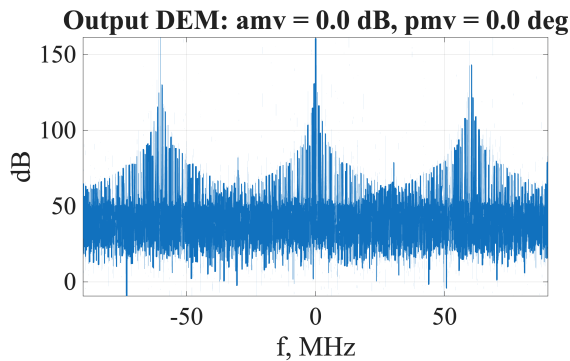
Рис. 14 — Идеальные квадратуры
