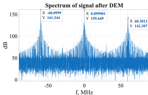
Рис. 9 — Спектр на выходе DEM
