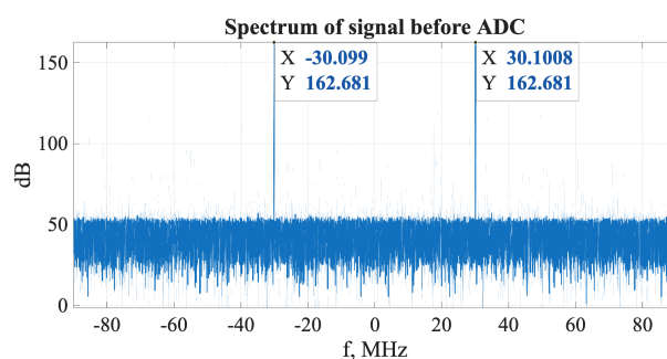
Рис. 3 — Спектр входного сигнала
