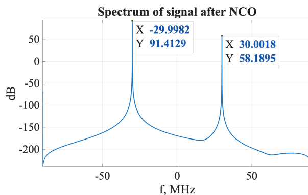
Рис. 7 — Спектр сигнала ЦГ
