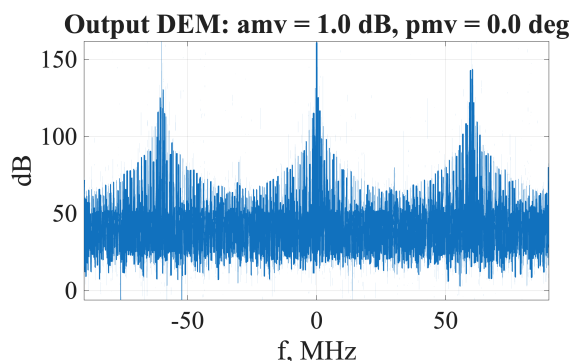
Рис. 16 — Амплитудный разбаланс (1 дБ)
