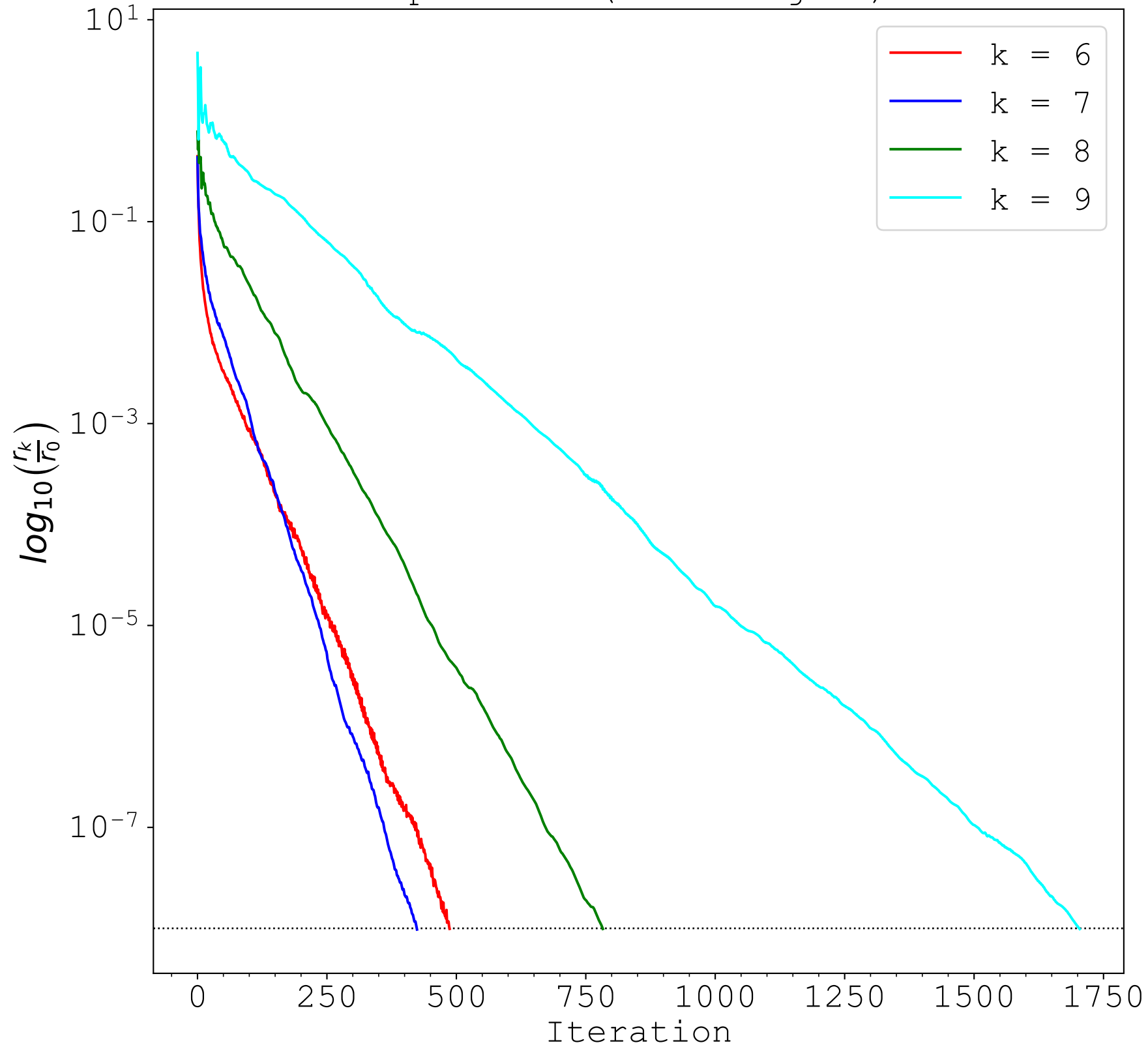
Sparse CG (no multigrid)
