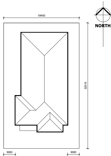
3 Site 1 : 200
