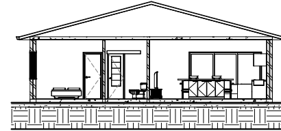
2 Section B-B 1 : 100
