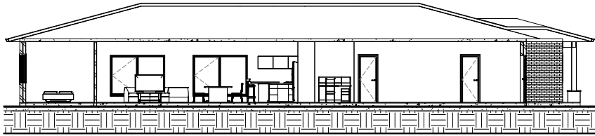
1 Section A-A 1 : 100
