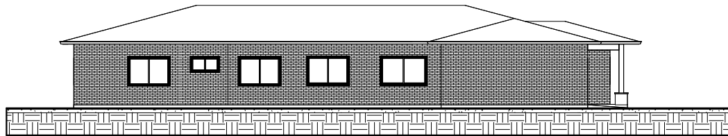
2 West 1 : 100
