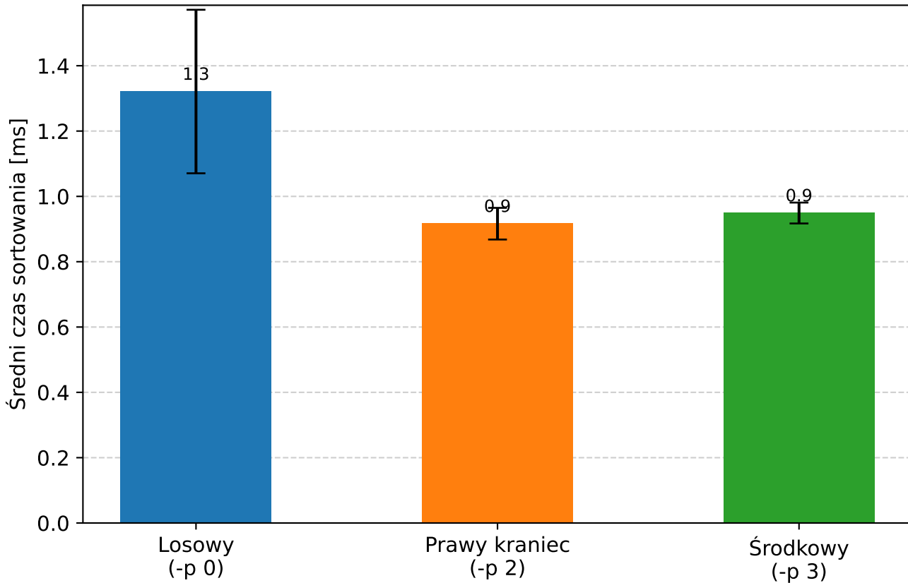
QuickSort: strategie wyboru pivota (n = 25 000, dane losowe, tablica, int)
