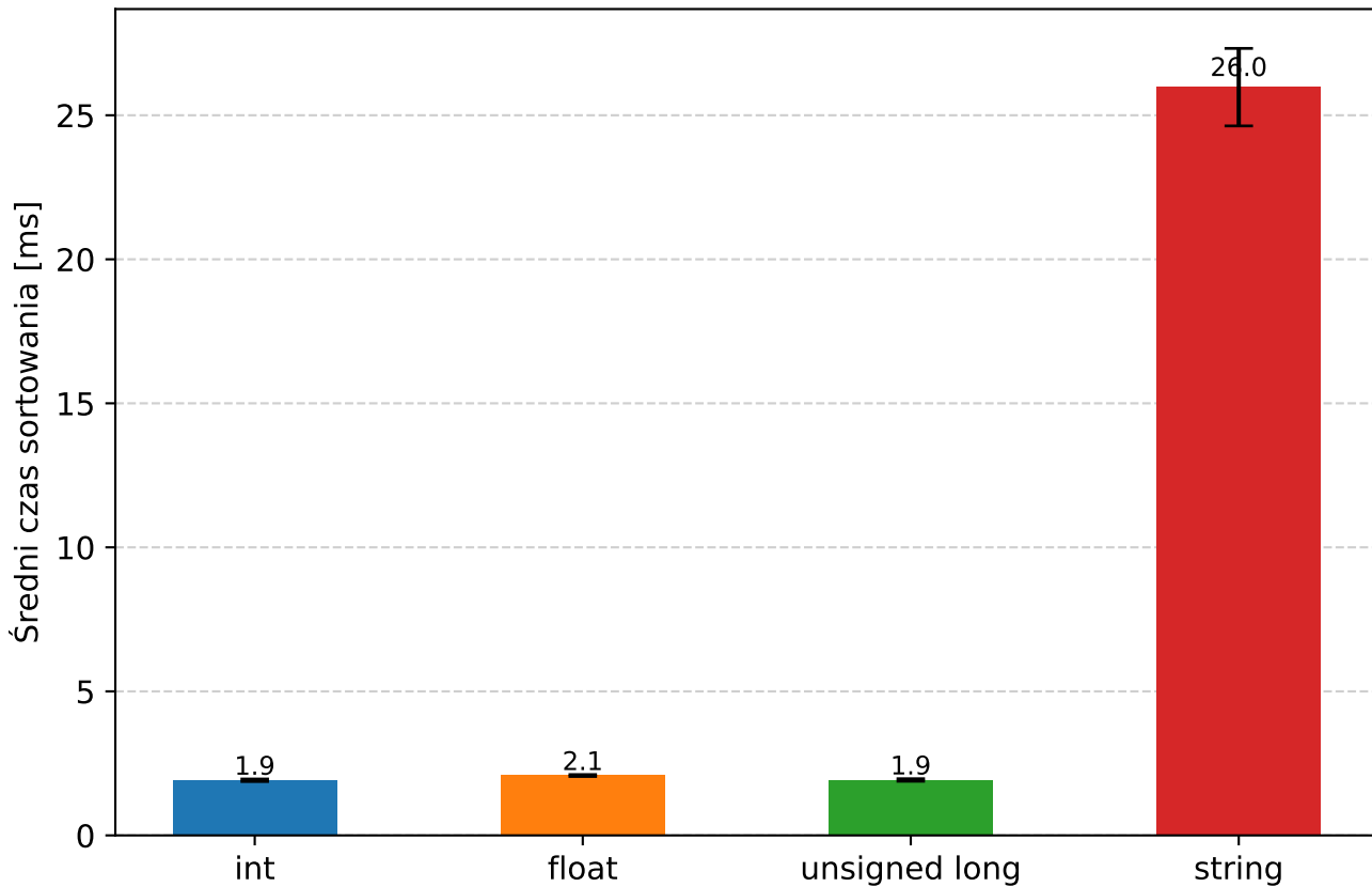
Badanie C: wpływ typu danych (QuickSort, pivot prawy, n = 25 000, tablica, rozkład losowy)
