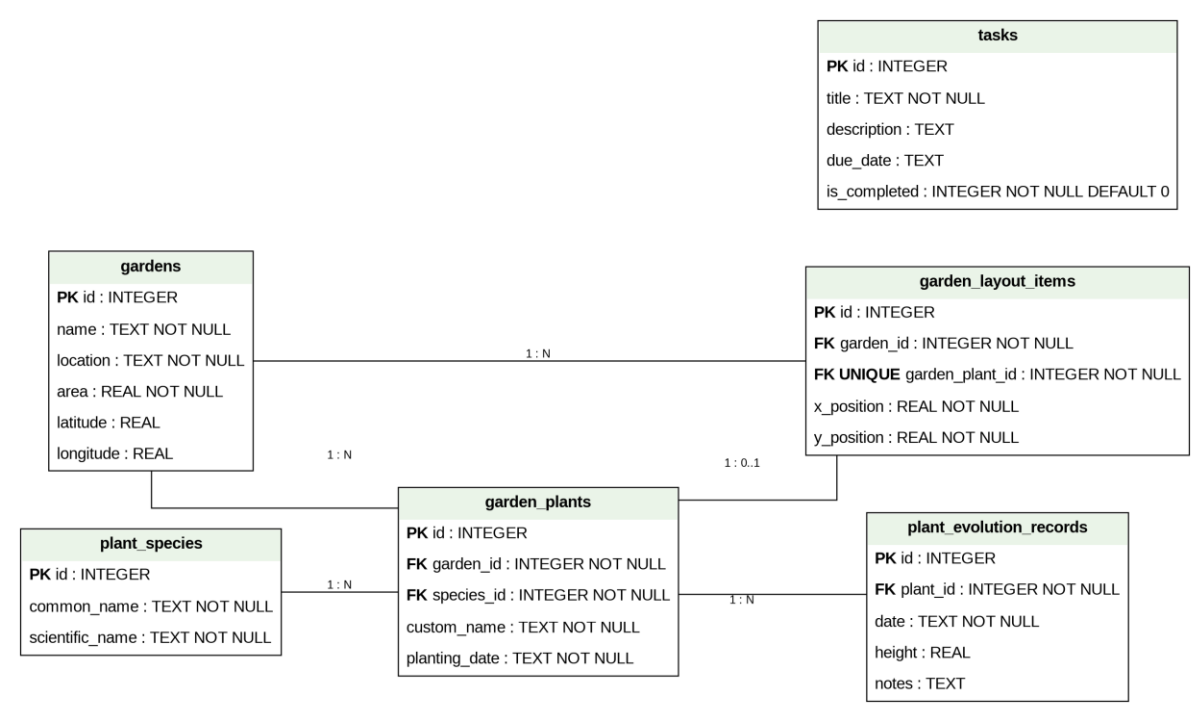
Figura 2. Diagrama entidade-relación do esquema físico final, versión 6.
