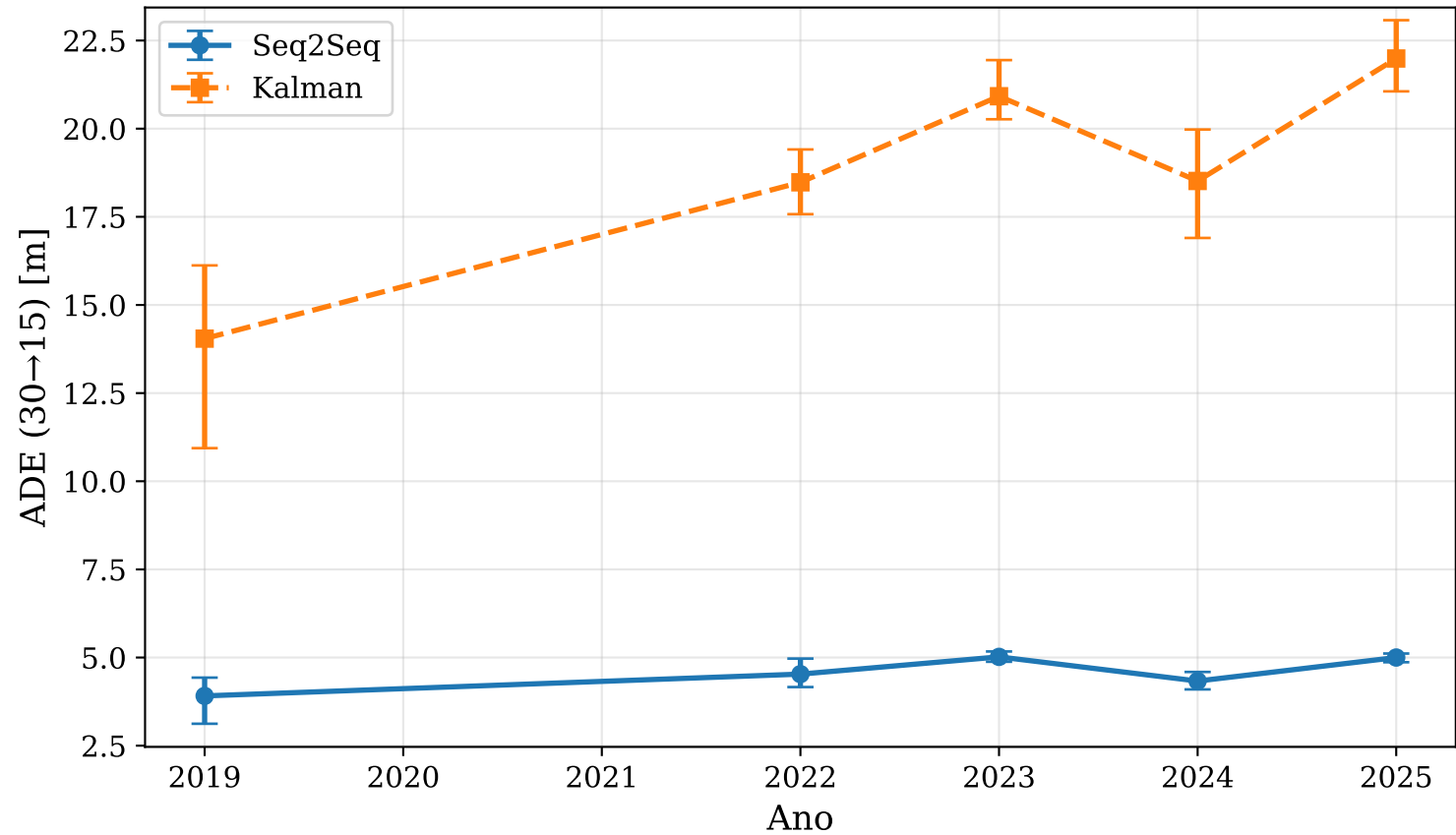
ADE por Ano — Seq2Seq vs Kalman (IC bootstrap)
