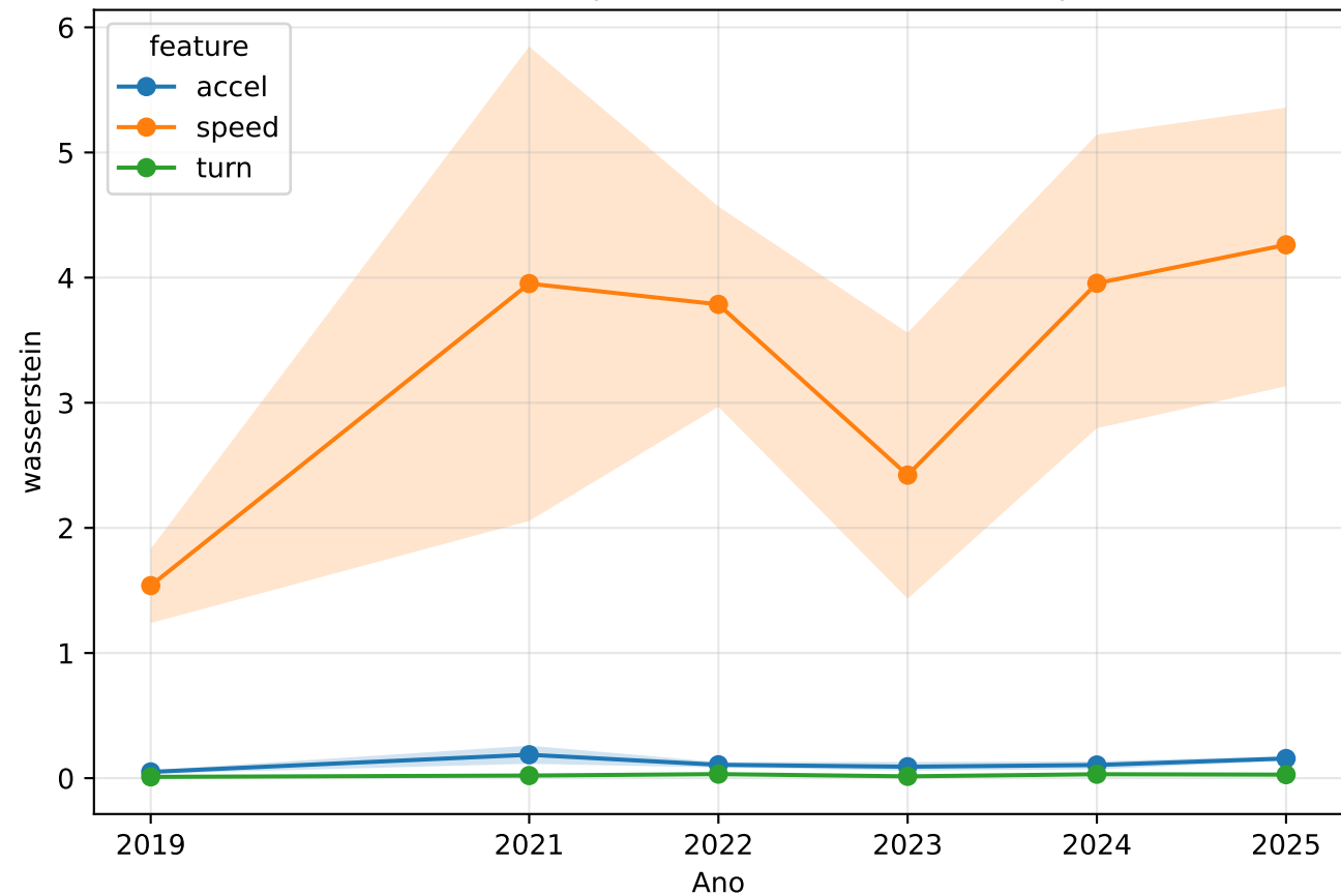
WASSERSTEIN por ano (IC95% via bootstrap)
