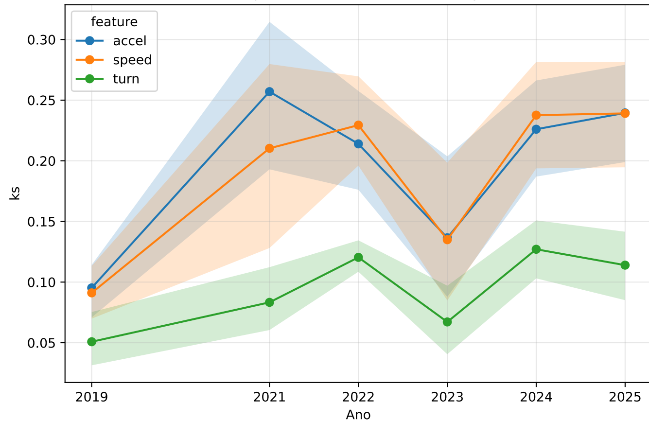
KS por ano (IC95% via bootstrap)
