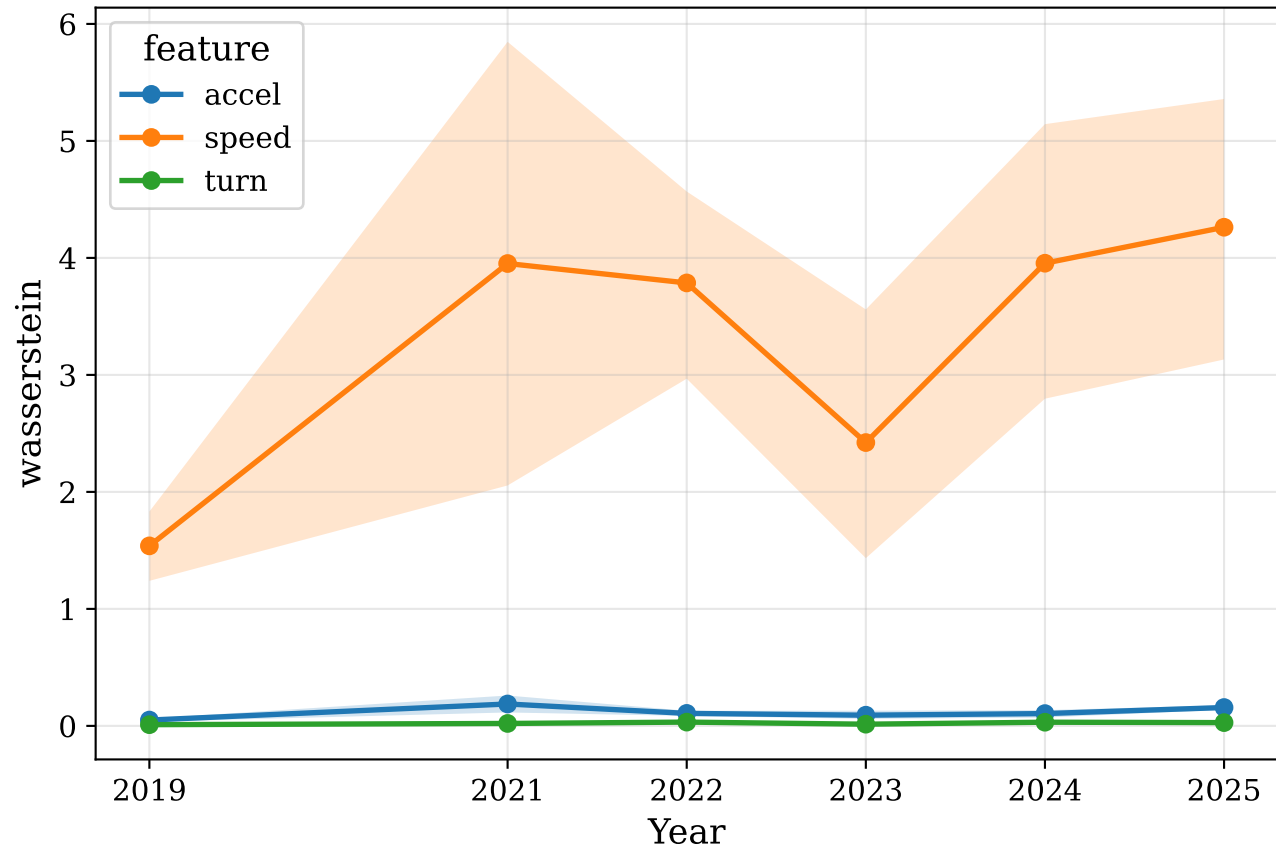
WASSERSTEIN per year (95% bootstrap CI)
