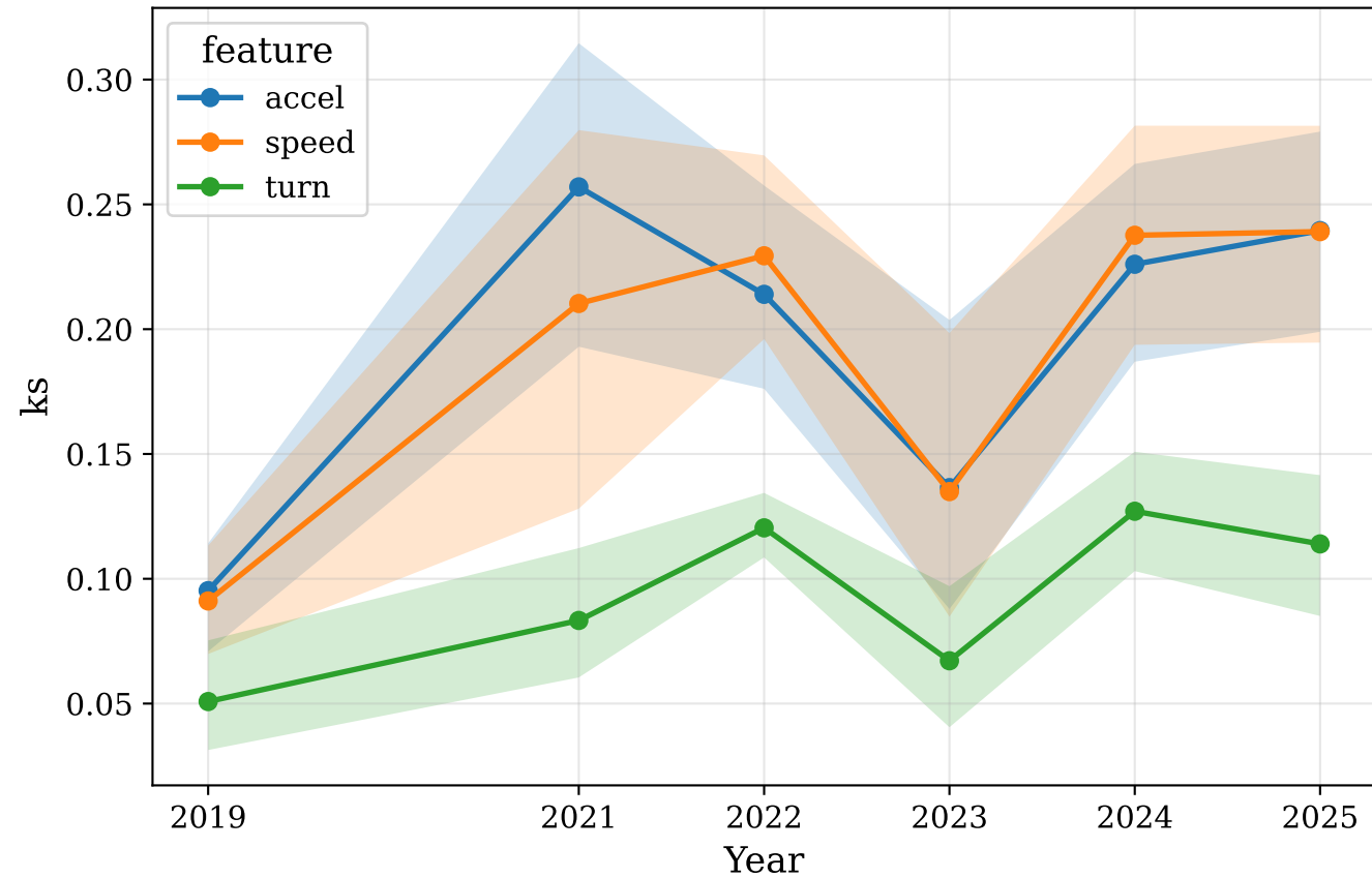
KS per year (95% bootstrap CI)
