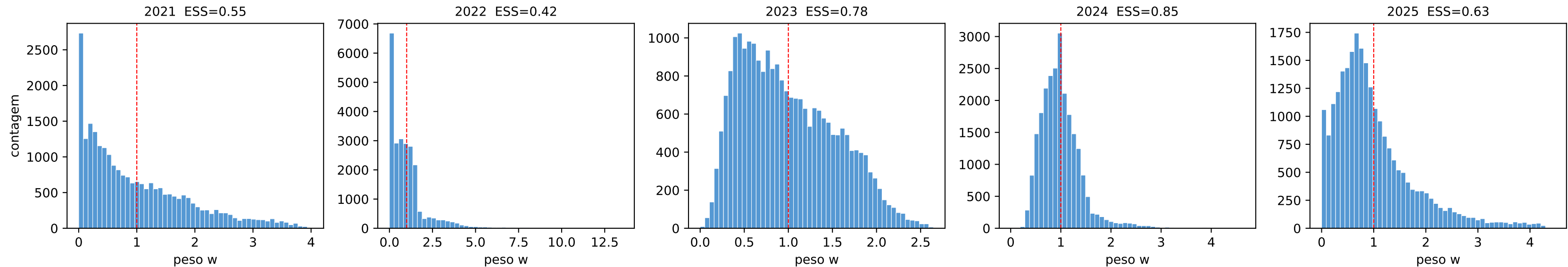
Distribuição dos pesos p_{2019}(x)/p_y(x) por ano
