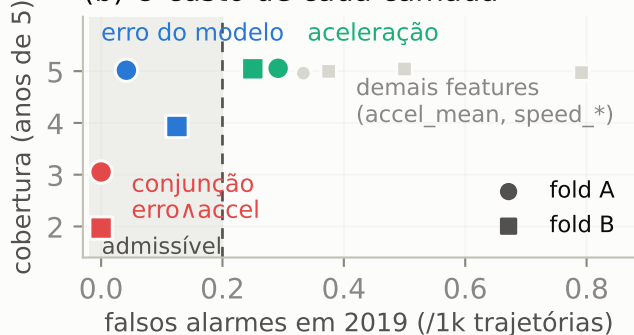
(b) O custo de cada camada
