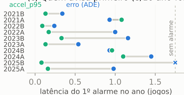
(c) Quem avisa primeiro (8/10 ano-folds)
