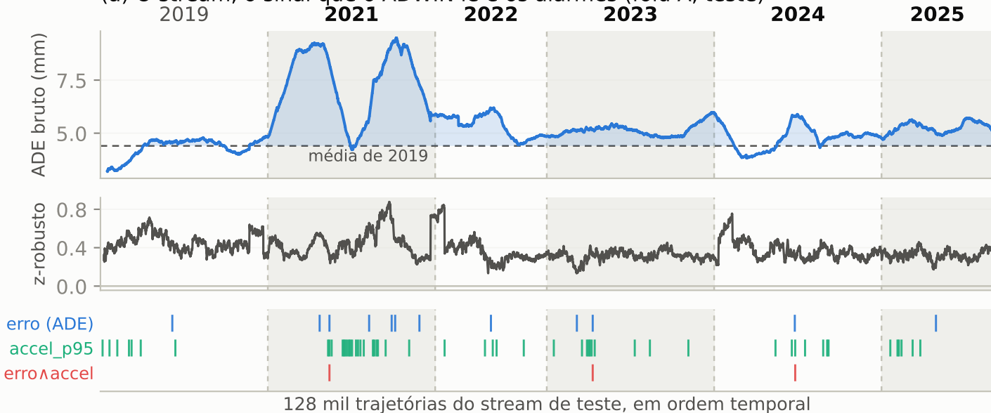
(a) O stream, o sinal que o ADWIN lê e os alarmes (fold A, teste)
