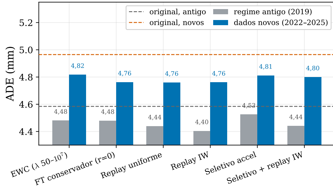
(b) ADE após adaptação
