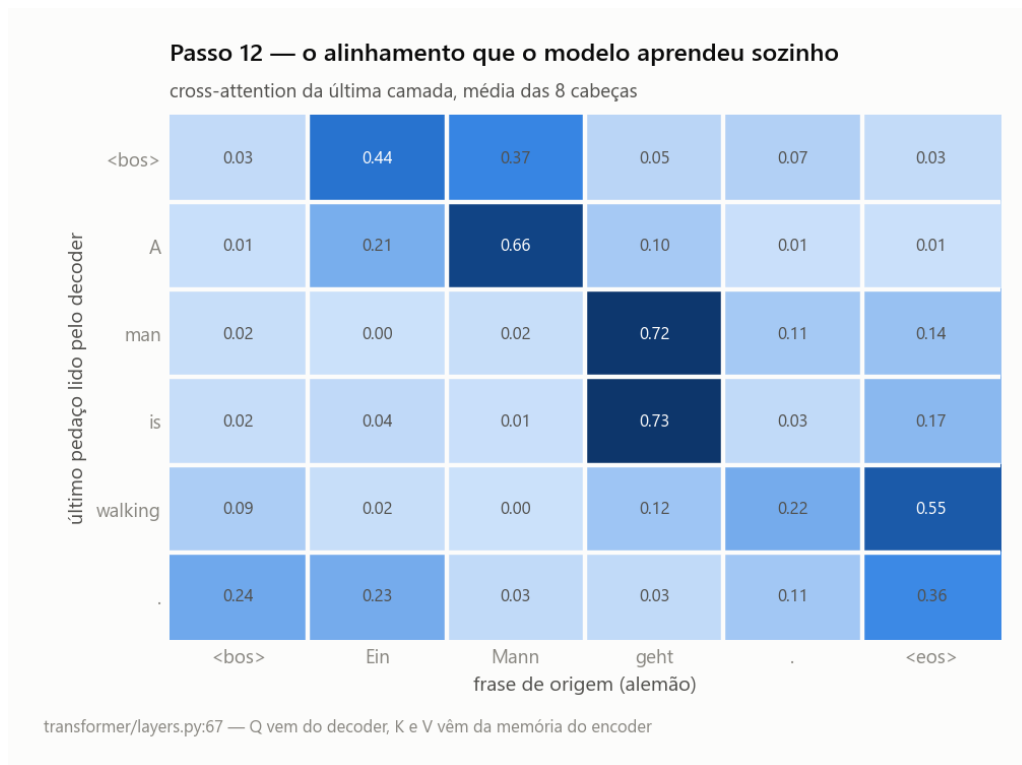
Figura 10: Alinhamento alemão→inglês extraído da cross-attention. Depois de ler “A”, o modelo olha para Mann ; ao gerar “is” e “walking”, olha para geht nas duas voltas — um alinhamento de uma palavra alemã para duas inglesas.
