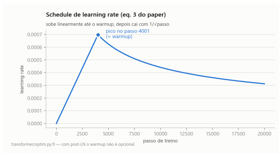
Figura 11: O cronograma de taxa de aprendizado, com o pico exatamente no fim do aquecimento.
