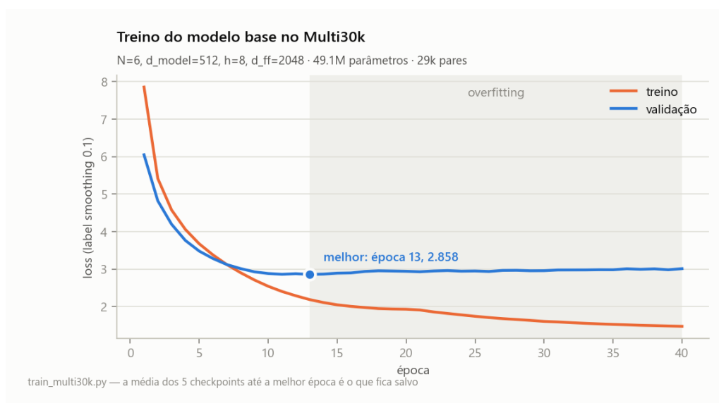
Figura 12: Treino no Multi30k. A partir da época 13 a perda de treino continua caindo enquanto a de validação sobe: o modelo passou a decorar.
