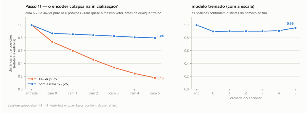
Figura 13: Distância média entre as posições ao longo das camadas do encoder, relativa à entrada. À esquerda, na inicialização, com e sem o amortecimento do ramo residual. À direita, o modelo treinado.
