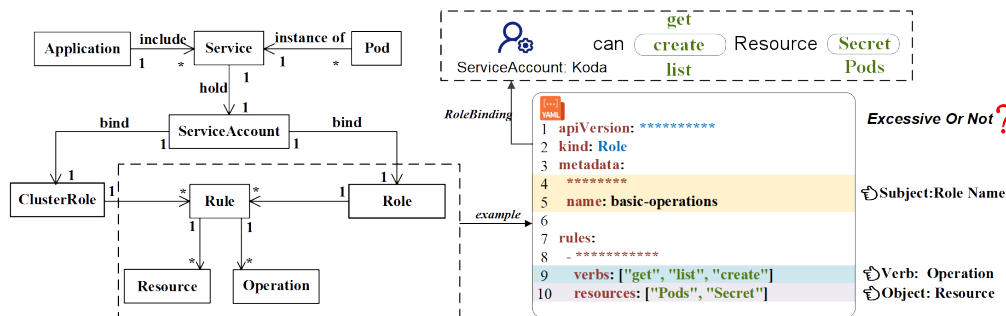
图 2-4 Kubernetes RBAC 权限配置 YAML 文件示意 [10]
