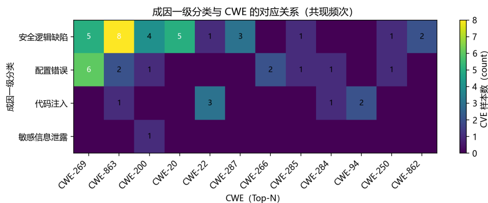
图 3-3: 成因一级分类与 CWE 的对应关系（Top CWE 共现频次热力图）
