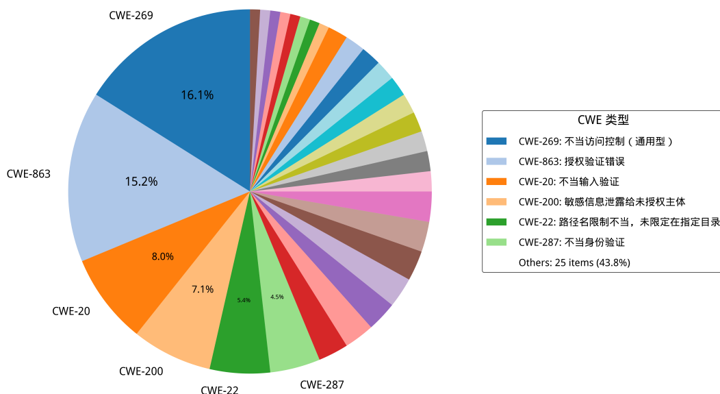
图 2-2: Kubernetes 权限提升 CVE 对应的 CWE 类型占比
