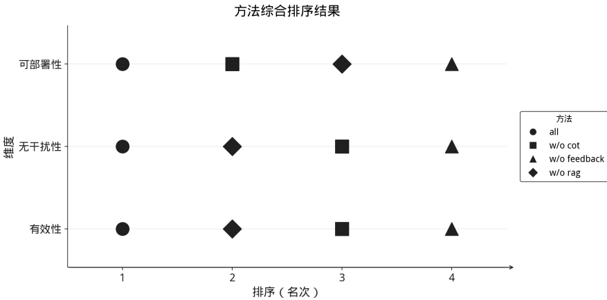
图 5-1: 方法配置在三个维度上的排名对比
