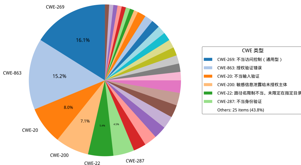
图 3-4: Kubernetes 权限提升 CVE 对应的 CWE 类型占比
