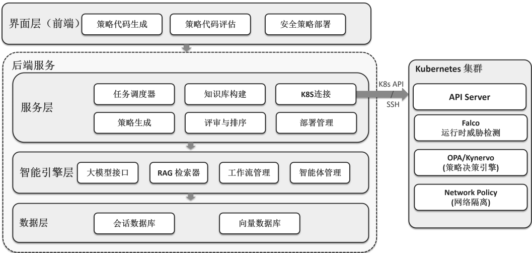
图 4-2 系统总体架构图
