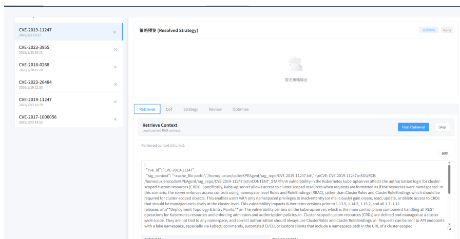
图 4-10: 检索增强（RAG）模块检索结果展示
