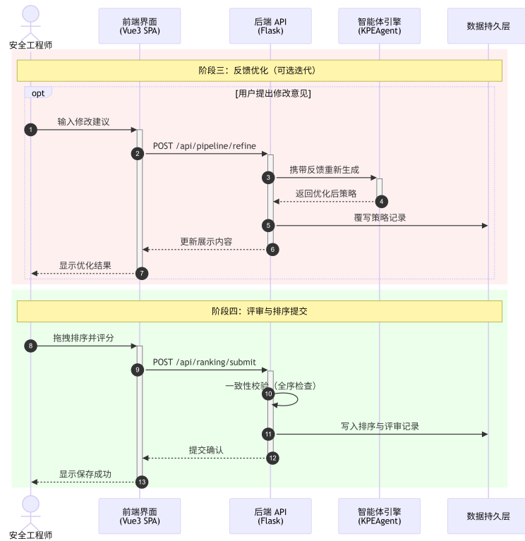
图 4-5: 反馈优化与评审排序的交互时序（UML 时序图）
