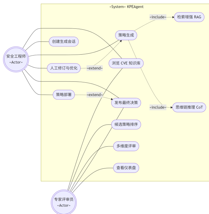
图 4-1: 系统用户角色与核心用例 (UML 用例图)
