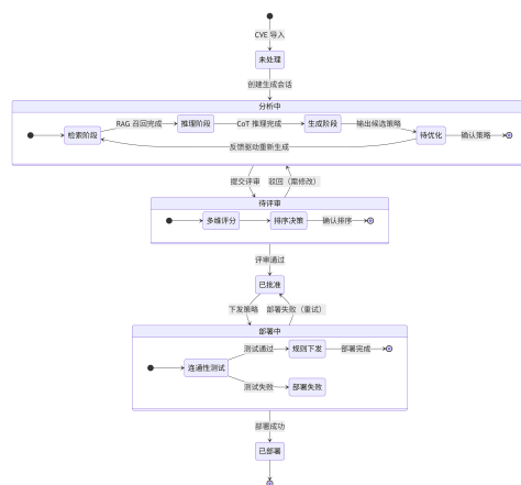
图 4-7: CVE 漏洞处置生命周期状态图 (UML 状态图)
