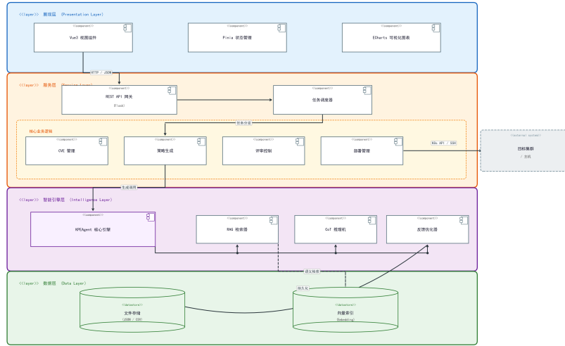
图 4-2: 系统总体架构与分层设计 (UML 组件图)
