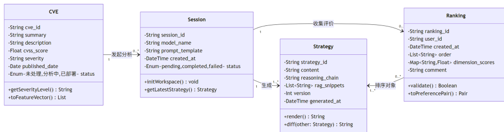
图 4-6: 系统核心实体类图（UML 类图）
