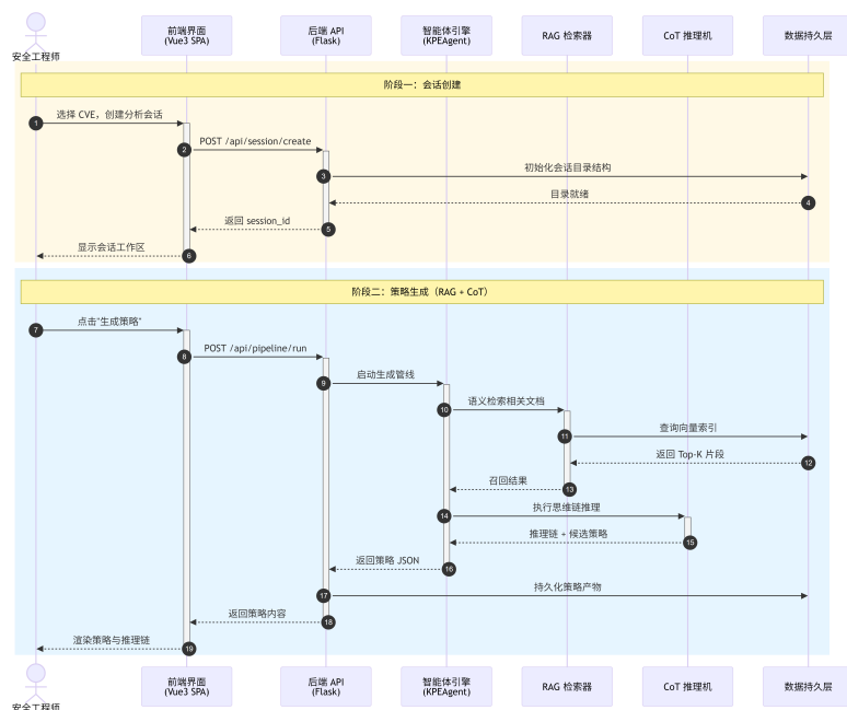
图 4-4: 会话创建与策略生成的交互时序（UML 时序图）
