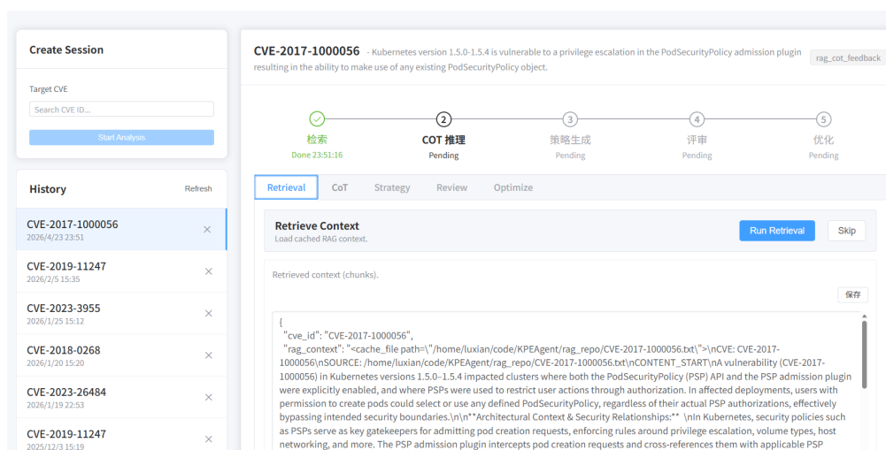
图 4-9 安全上下文检索结果展示
