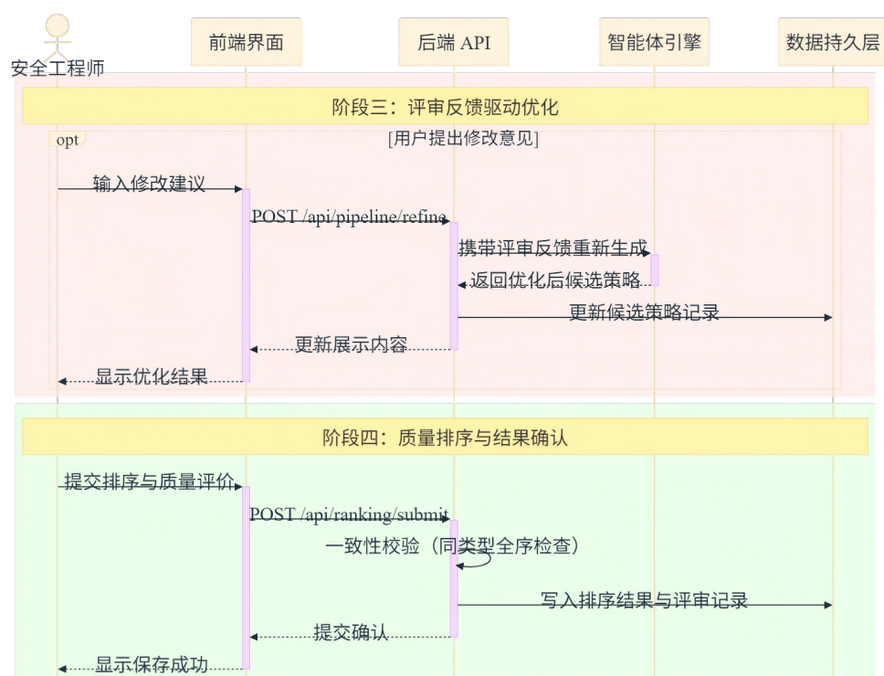
图 4-6 评审反馈优化与质量排序确认时序
