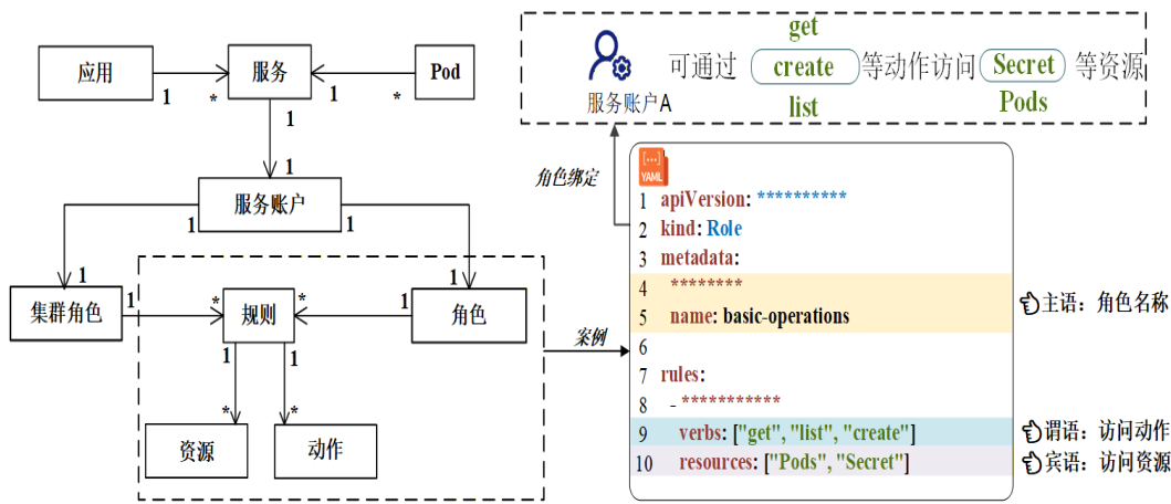
图 2-4 K8s RBAC 权限配置 YAML 文件示意 [1]
