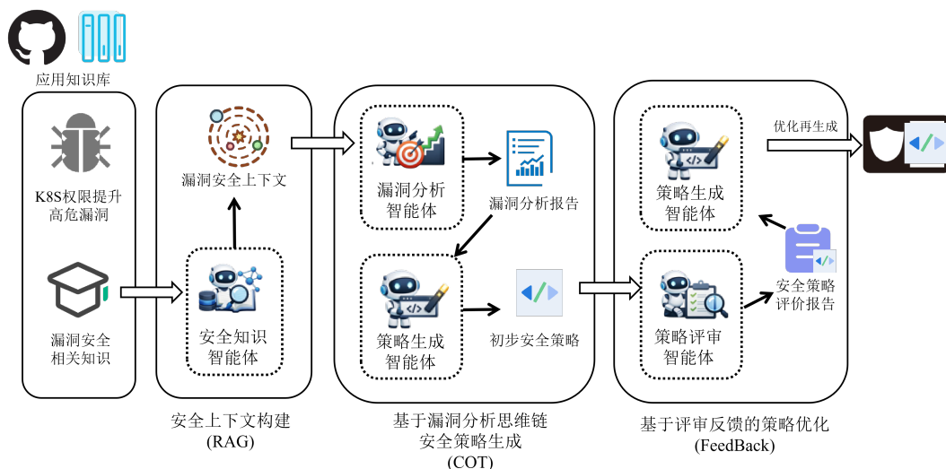
图 3-4 基于多智能体的安全策略生成与优化工作流
