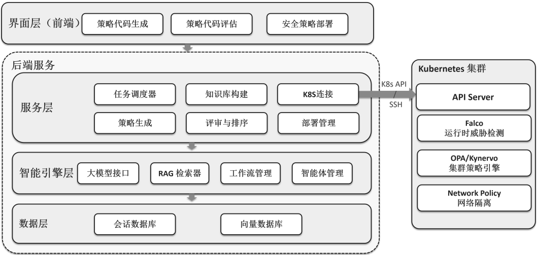
图 4-2 KPEDefense 支持工具总体架构图
