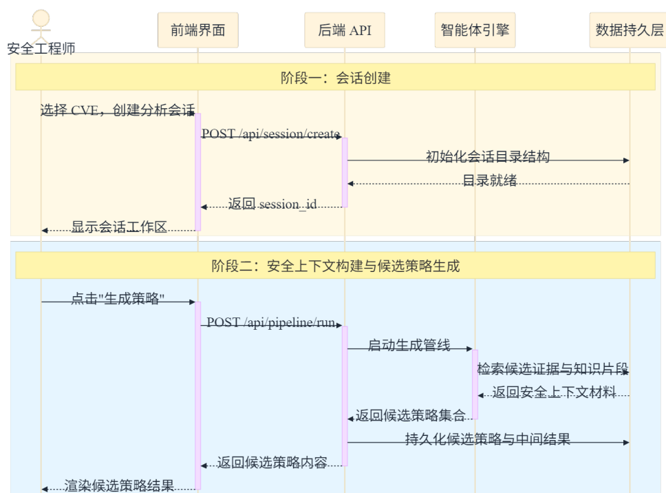
图 4-5 会话创建与候选策略生成时序图
