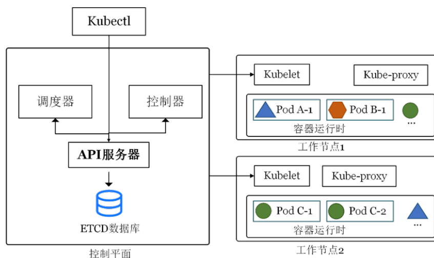
图 2-2 K8s 体系结构示意
