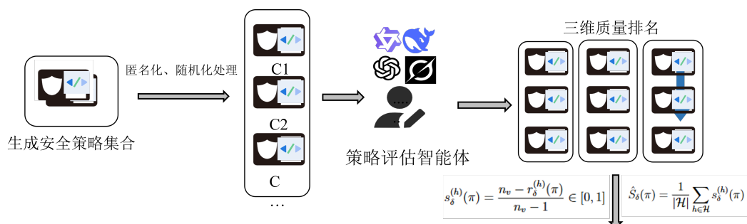
图 3-10 基于排名的多源模型三维质量评价方法
