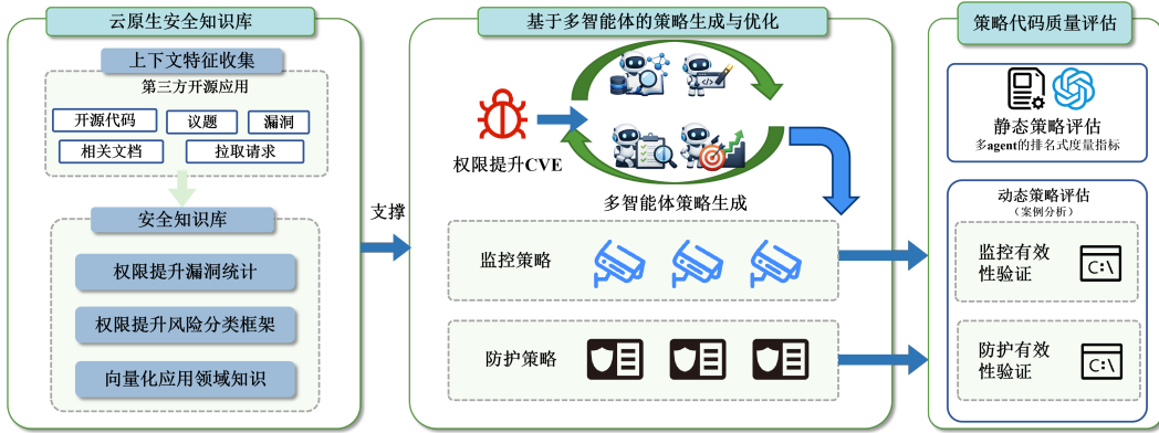
图 3-1 智能化漏洞监控与防护安全策略生成方法总体框架
