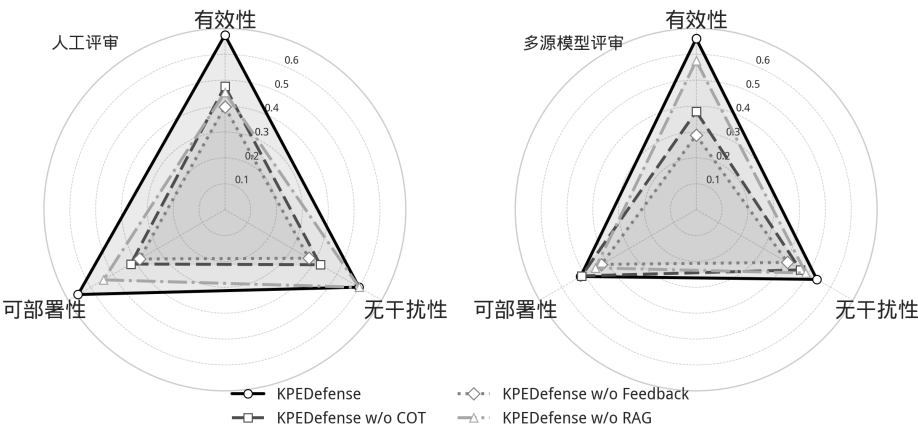
图 5-1 人工评估与多源模型评估下不同方法配置策略质量三维度雷达图对比
