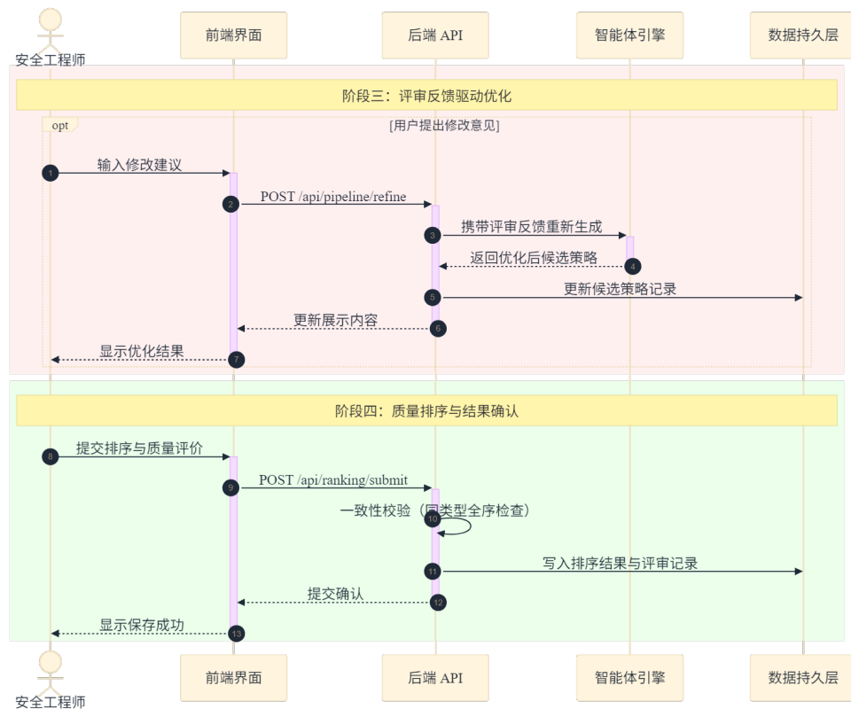
图 4-6 评审反馈优化与质量排序确认时序
