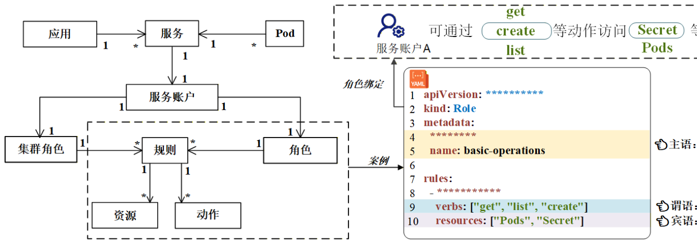
图 2-4 K8s RBAC 权限配置 YAML 文件示意 [1]
