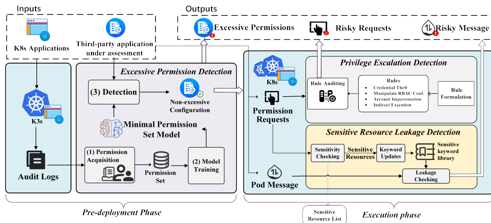
图 2-8: KubeGuard 方法框架图 [10]
