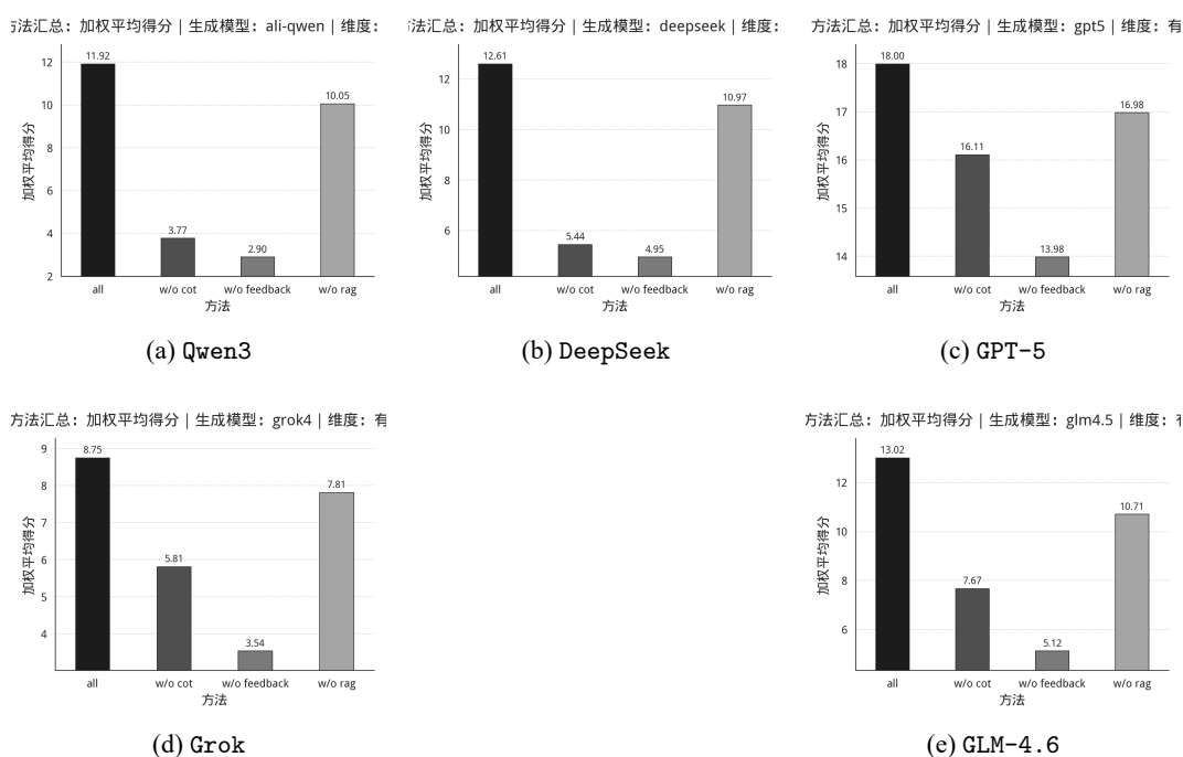
图 5-4: 有效性维度下, 不同生成模型的工作流贡献结构对照 (3+2 网格)。
