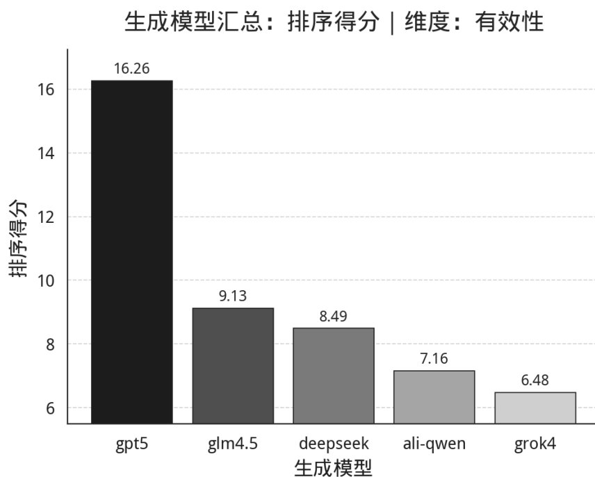
图 5-3: 有效性维度下, 不同生成模型的平均排名式评分结果 (跨评审者汇总)。
