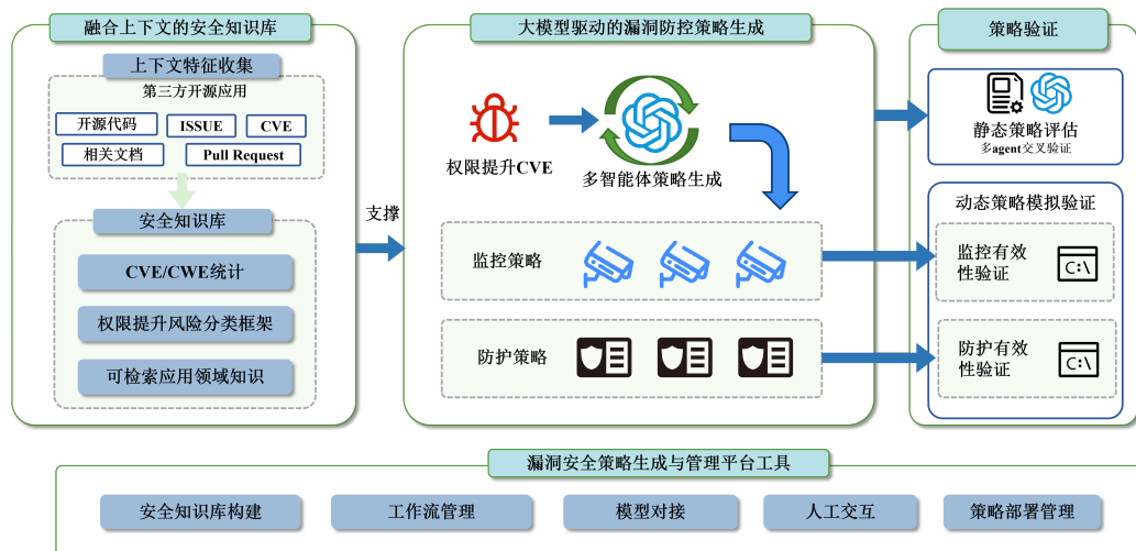
图 1-2: 基于大语言模型的多 Agent 漏洞临时防控总体框架
