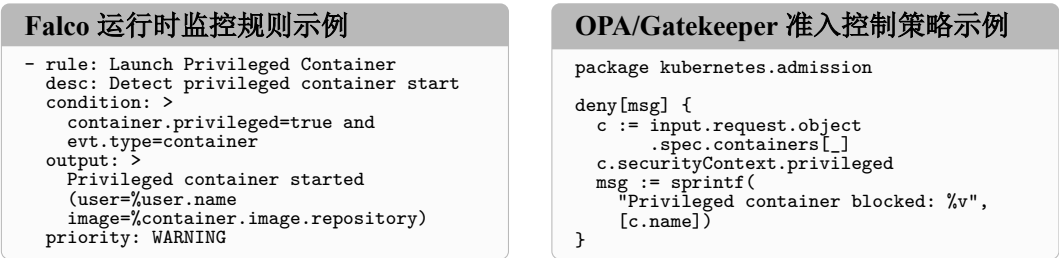
图 2-6 Falco 运行时监控规则与 OPA/Gatekeeper 准入控制策略示例
