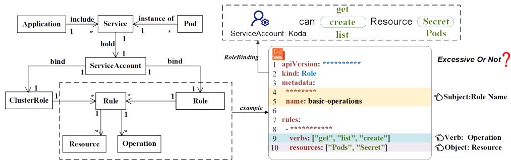
图 2-4 K8S RBAC 权限配置 YAML 文件示意 [2]
