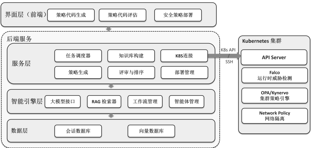
图 4-2 KPEDeDefense 支持工具总体架构图
