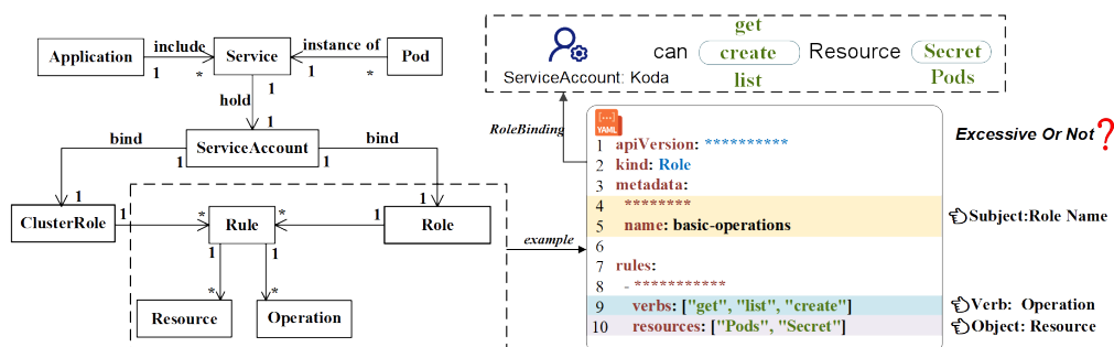
图 2-3: Kubernetes RBAC 权限配置 (YAML) 示意 [?]
