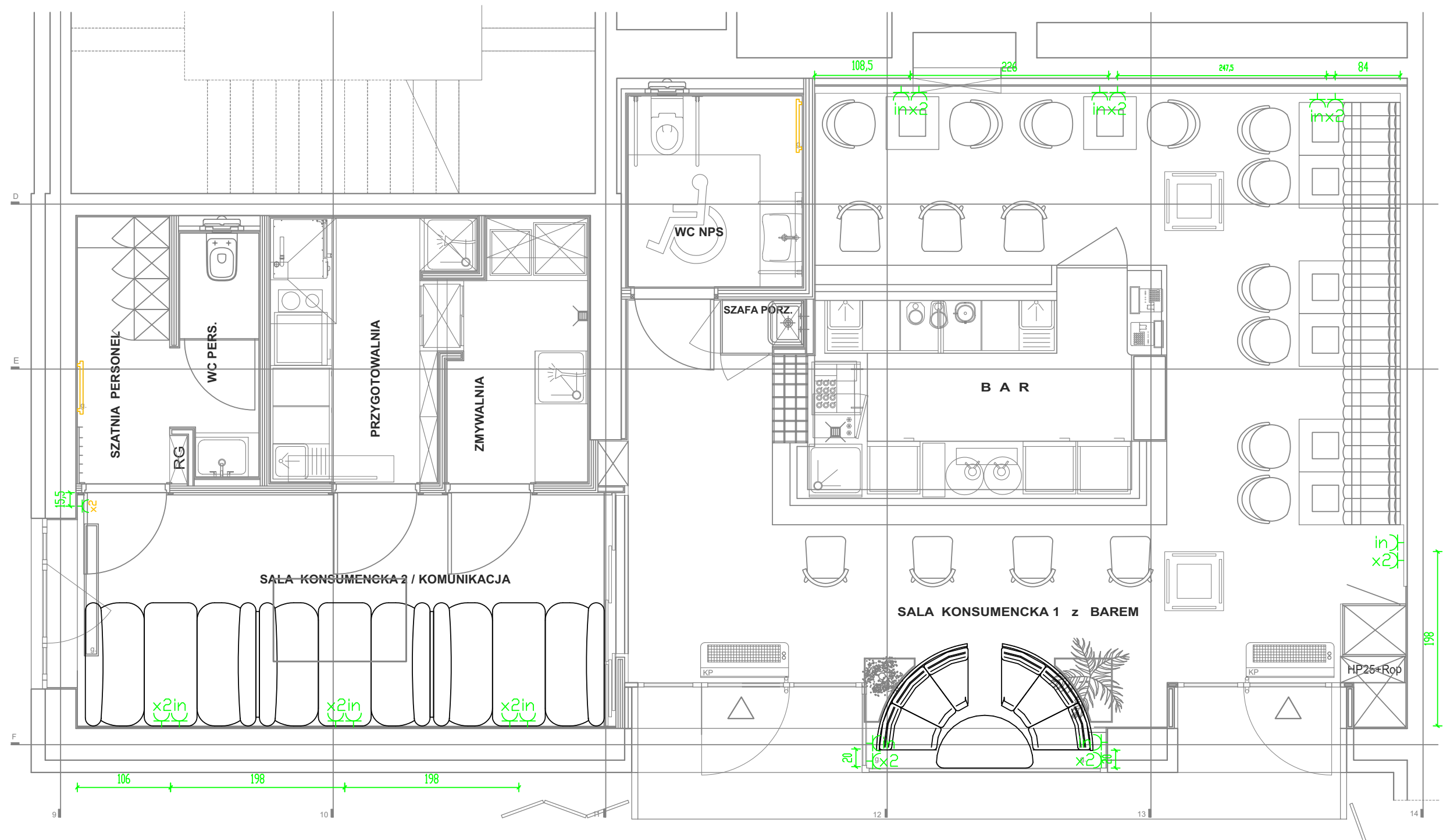
Część elektryczna dla klientów - nowy projekt gniazda na wysokości 20cm od docelowej podłogi
