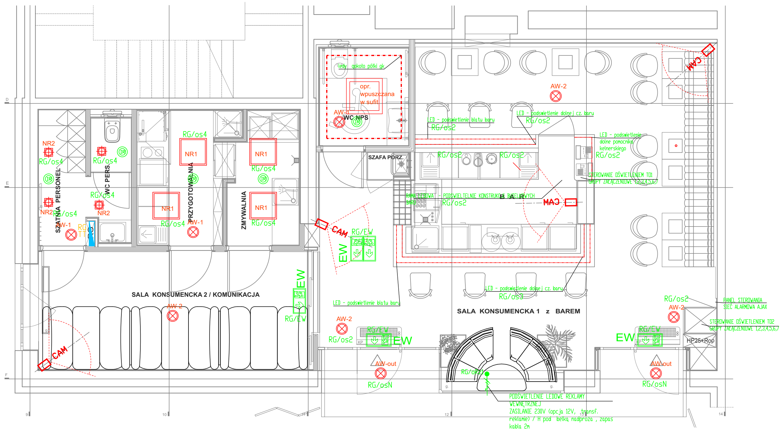
Część oświetlenia technicznego - pozostawiona z poprzedniego projektu
