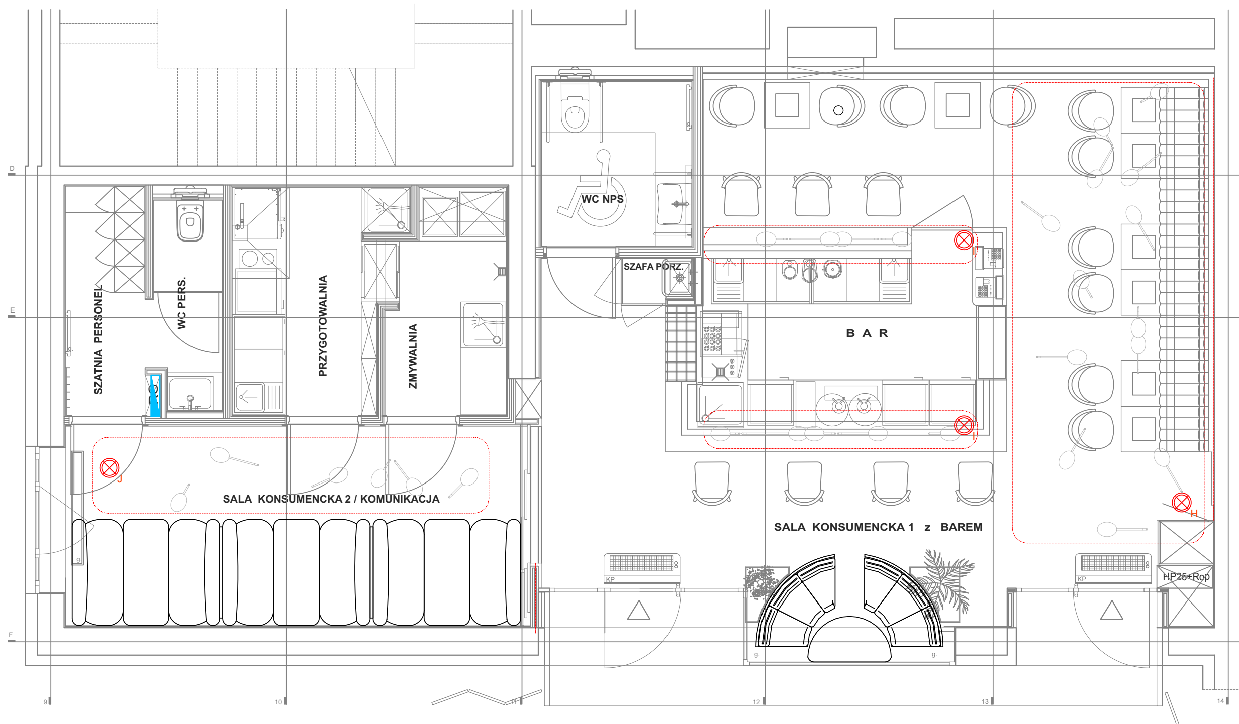
sugerowane rozmieszczenie opraw dekoracyjnych i ich grupy
