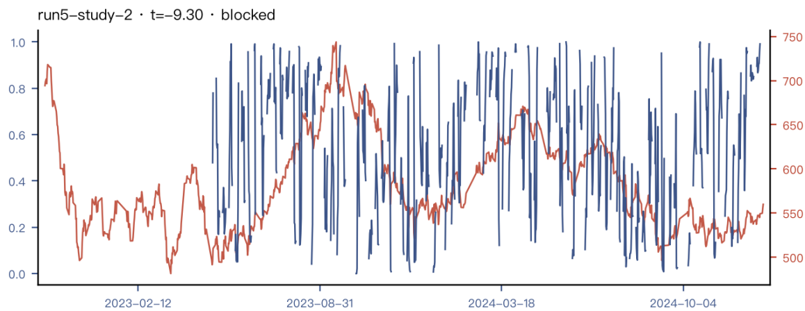
图 1：波动假象 run5-study-2 ( t = -9.30 )：信号与价格。该信号实为已实现波动的函数，与目标同源。
