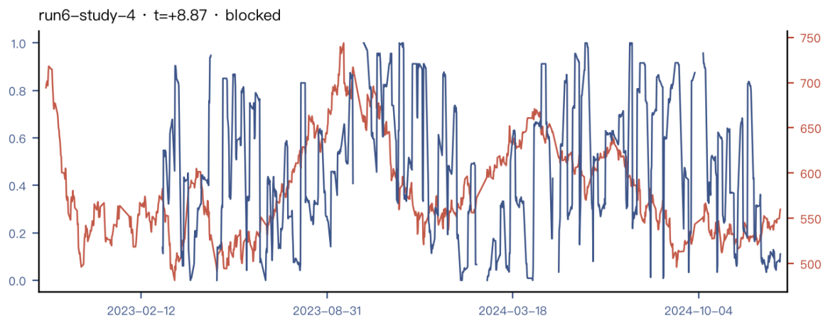
图 2: 波动假象 run6-study-4 ( t = +8.87 ): 信号与价格。该信号实为已实现波动的函数，与目标同源。
