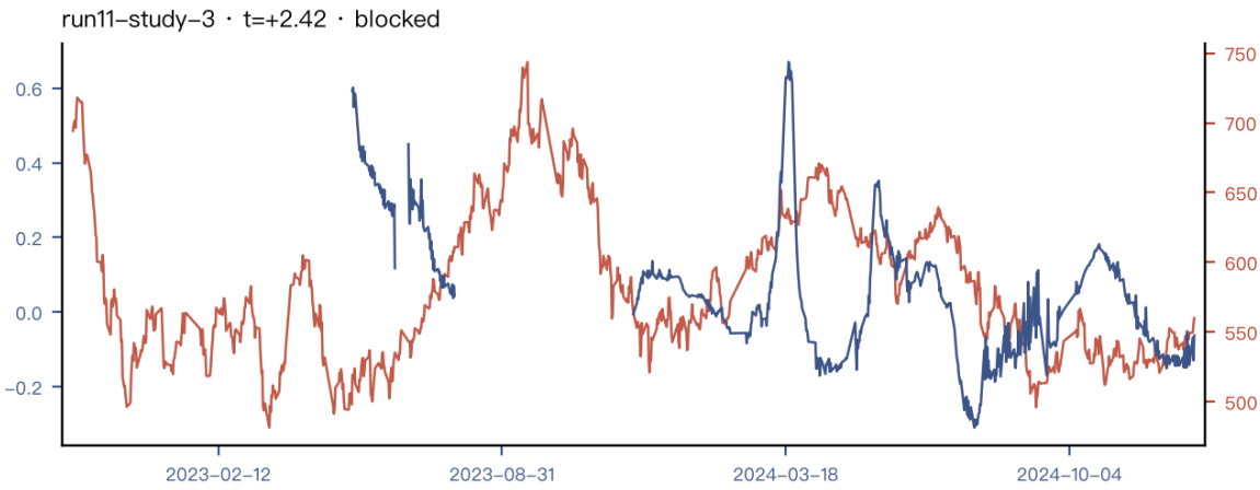
图 3: 唯一走完全流程的候选: 信号 (蓝, 左轴) 与 SC 收盘价 (红, 右轴)。信号由冻结规格在 discovery 决策网格上重新求值, 非回放存档。
