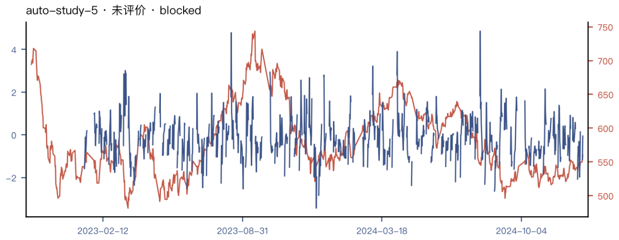
auto-study-5: rv_innovation_z_1d_vs_14d。有定义 835/1040 点。
