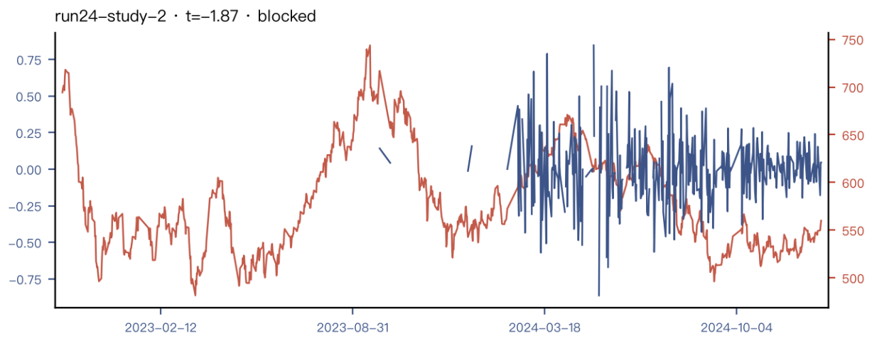
run24-study-2: pm_ukraine_strike_hazard_dev_evt_6h_vs_prior_1d_resid_brent_90d_fu。有定义 463/1040 点。
