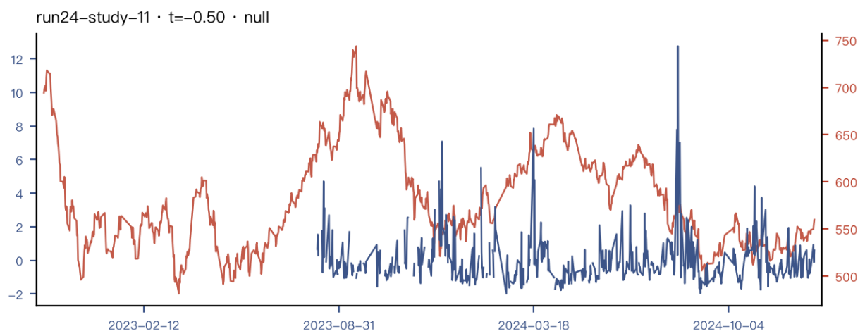
run24-study-11: pm_ukraine_evt_arrival_crowding_over_a_baseline_resid_own_rv_12h_30d_90d_bu。有定义 604/1040 点。
