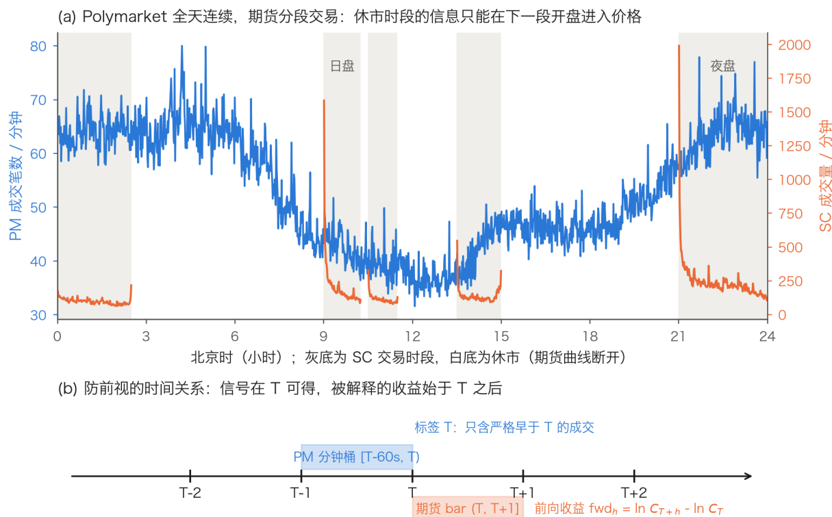
图 1: (a) Polymarket 登记市场成交笔数与 SC 成交量的日内分布（北京时，125 天均值；灰底为 SC 交易时段，休市后期货曲线断开）。(b) 防前视的时间关系：分钟桶右端标签使信号严格早于被解释的收益。
