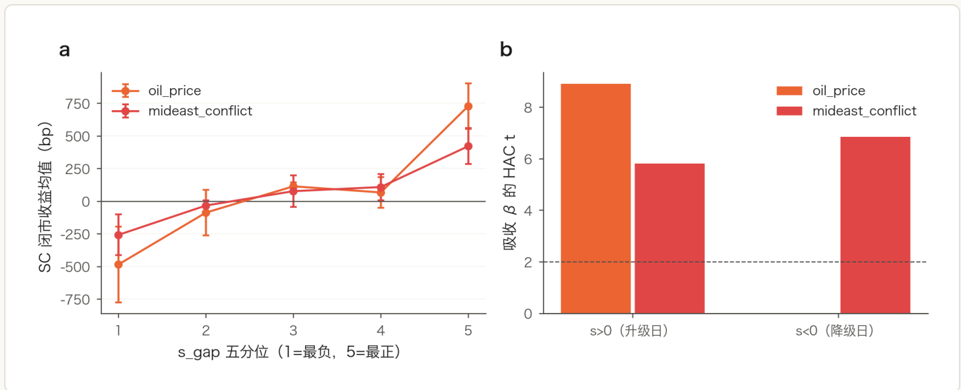
(a) s_gap 五分位组的 SC 闭市收益均值 \pm 标准误：单调；(b) 升级日 vs 降级日分别估计的吸收 \beta 的 HAC t 。
