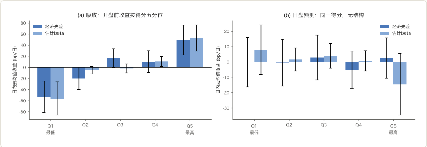
(a) 吸收：开盘前收益随暴露度五分位近单调上行（Q1 约 -53/-56 bp/日，Q5 约 +49/+53 bp/日，误差线为 HAC 95% CI）；(b) 日盘预测：同一得分五分位全部与零不可分。
