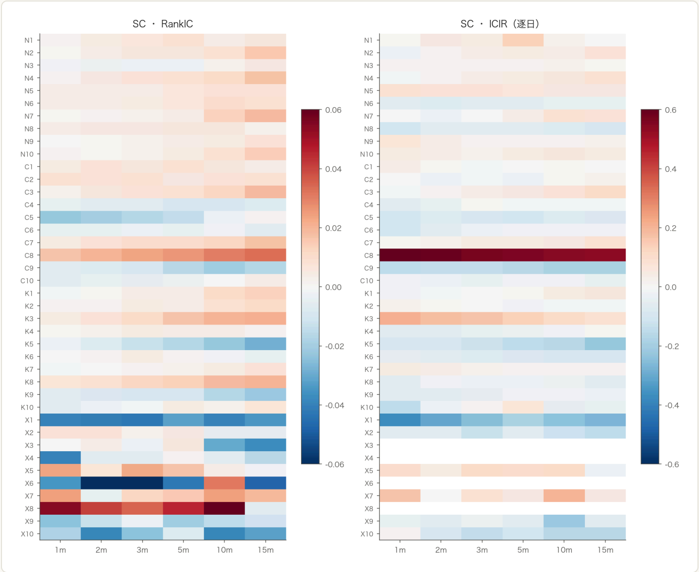
SC 的 40 信号 \times 6 视界 RankIC 与 ICIR 热图（红 = 正、蓝 = 负；ICIR 空缺见下文条件）。
