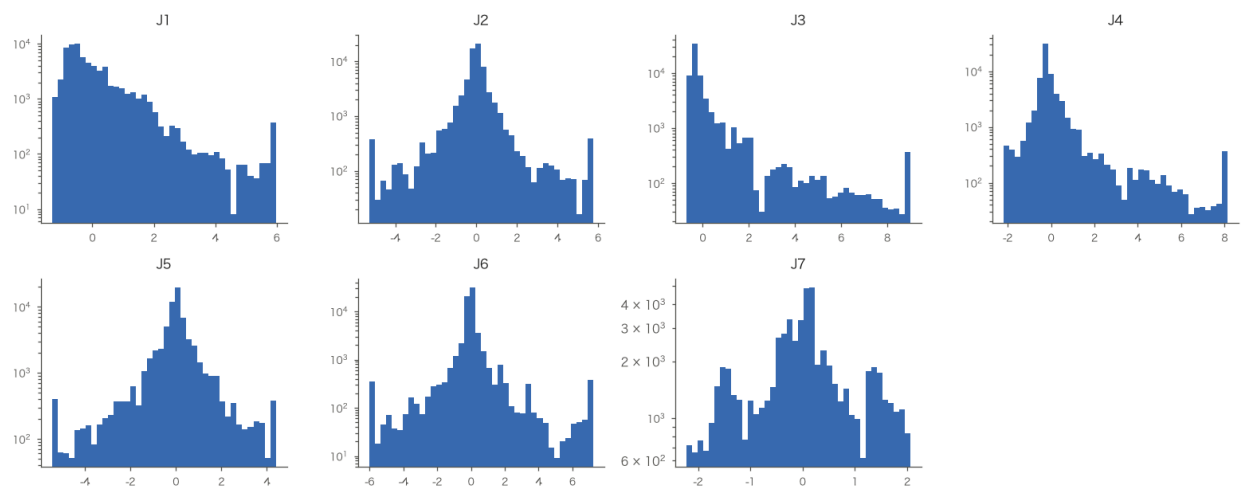
图 41 J 族因子非零取值分布 (SC, 滚动 z 后, 截尾 [0.5%, 99.5%], 对数频数轴)。J 族统计量 (均值 / 中位数 / 标准差 / 偏度 / 峰度 / 非零频率) 连同 40 信号一并收录于 signal_stats_ext.parquet (47 信号 \times 5 品种)。
