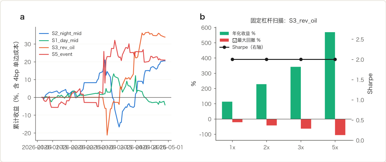
图 25 (a) 四个代表性策略的净值曲线 (含 4bp 单边成本); (b) 固定杠杆扫描: Sharpe (黑线, 右轴) 对杠杆不变, 收益 (绿) 与回撤 (红) 同比放大。
