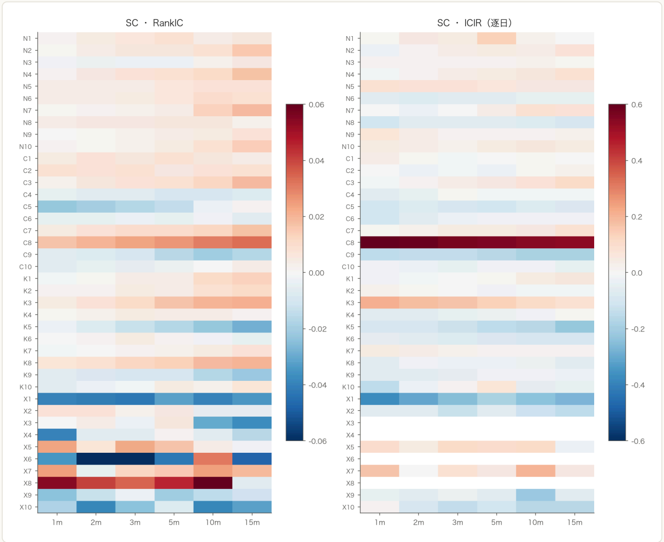
图 42 SC 的 40 信号 × 6 视界 RankIC 与 ICIR 热图（红 = 正、蓝 = 负；ICIR 空缺见下文条件）。
