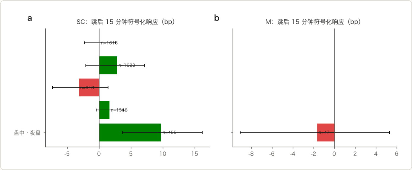
SC 与 M 的跳后 15 分钟符号化响应（按时段，自助 CI）。
