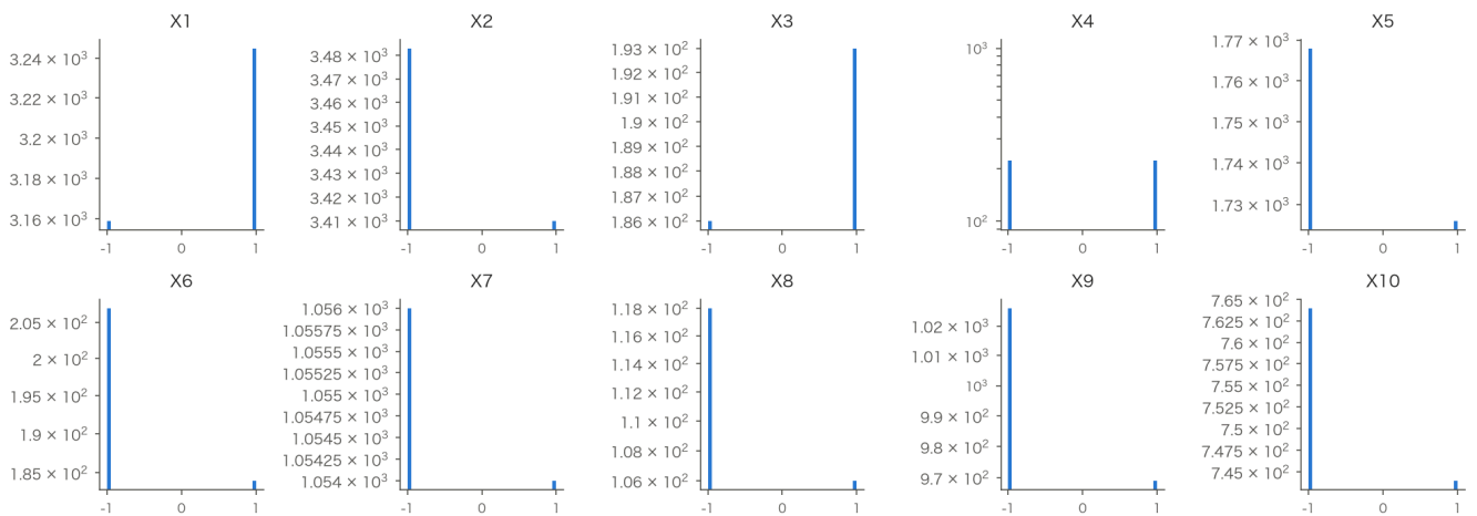
X 族信号非零取值分布 (SC, 截尾 [0.5%, 99.5%], 对数频数轴)。X 族取值集中在 \pm 1 (签名离散型)。
