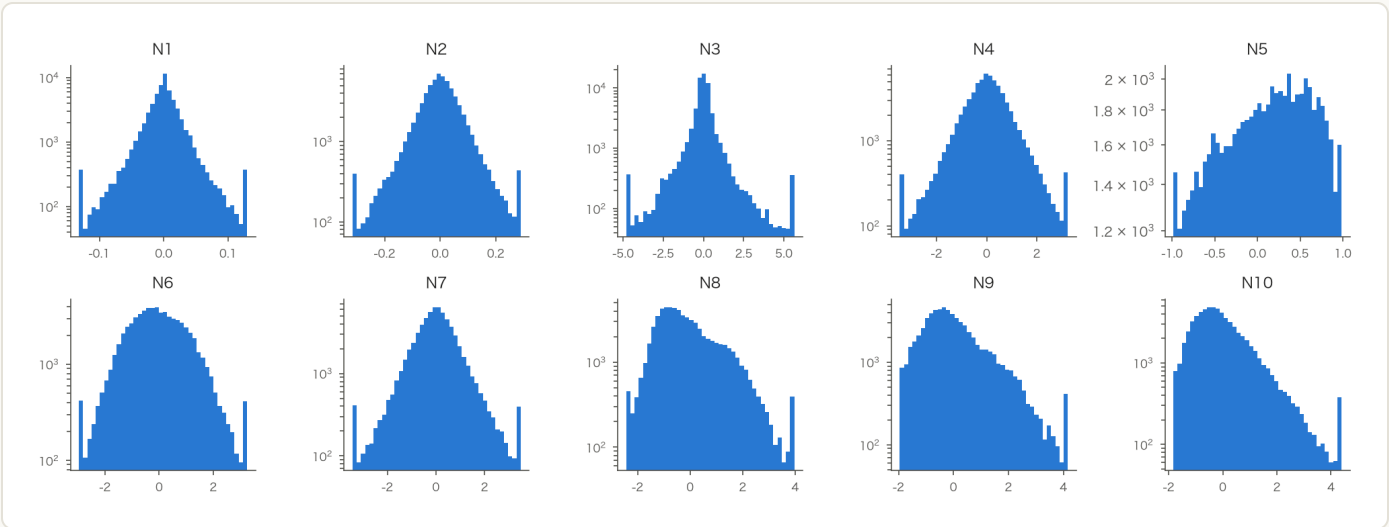
N 族信号非零取值分布（SC，截尾 [0.5%, 99.5%]，对数频数轴）。
