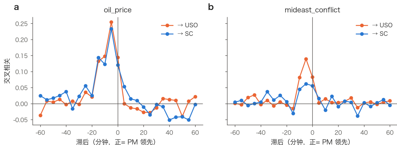
(a) oil_price、(b) mideast_conflict 主题 innovation 对 USO（橙）与 SC（蓝）的 \pm 60 分钟交叉相关：正滞后侧均无领先。
