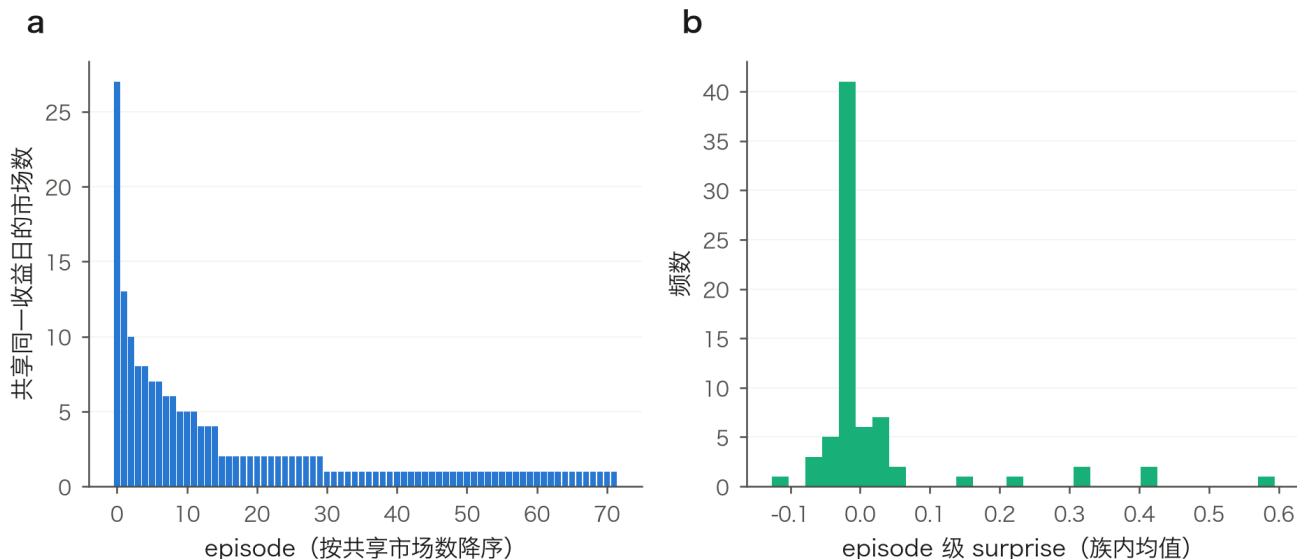
(a) mideastxSC 各 episode 共享同一收益日的市场数（最大 27）——伪重复的直观呈现；(b) episode 级 surprise 分布：SD 0.12、IQR 0.021， |s|>0.2 的事件批次仅 6 个——即便功效门槛放行，系数也几乎由这 6 天决定。
