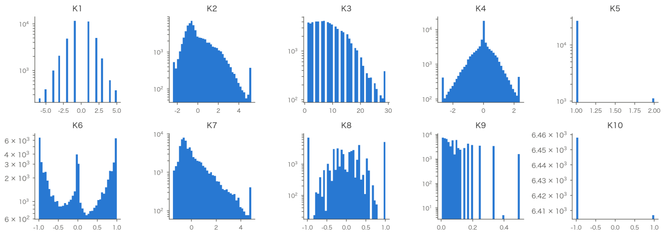
K 族信号非零取值分布 (SC, 截尾 [0.5%, 99.5%], 对数频数轴)。
