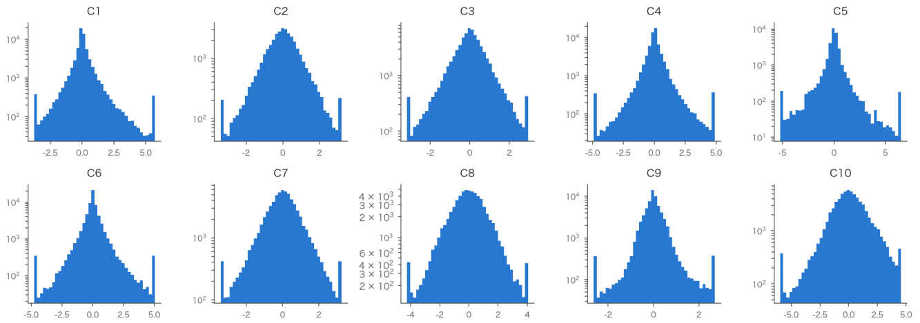
C 族信号非零取值分布 (SC, 截尾 [0.5%, 99.5%], 对数频数轴)。
