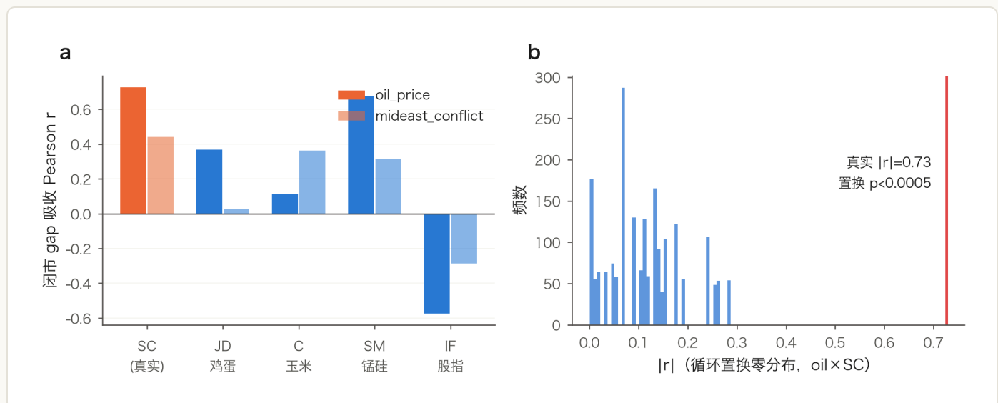
(a) 真实配对 (SC, 橙) 与四个安慰剂品种的闭市 gap 吸收：安慰剂不为零，揭示宏观共同因子；(b) oil×SC 的循环置换零分布与真实值 (红线)。
