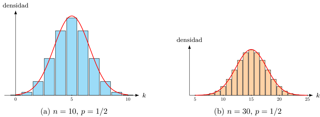
Figure 10: Distribución Binomial( n, 1/2 ) (barras) y la aproximación normal N(np, np(1-p)) del teorema de De Moivre–Laplace (curva roja). La aproximación mejora al crecer n , tal como predice el Teorema ??.
