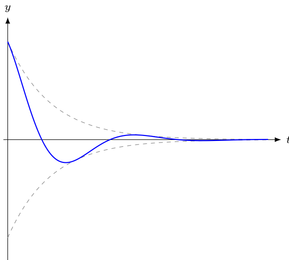
Figure 8: y(t) = e^{-t} \cos(2t) : la parte real de e^{(-1+2i)t} . Las envolventes \pm e^{-t} (gris punteado) muestran el amortiguamiento; el factor \cos(2t) , heredado de la parte imaginaria \pm 2i de la raíz, produce la oscilación.
