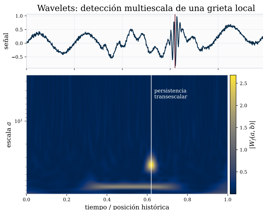
Figura 3: Lectura wavelet de una grieta local. Arriba aparece una señal histórica idealizada; abajo, un escalograma de coeficientes wavelet. La línea vertical marca un punto de condensación en el que varias escalas se alinean: no es sólo un pico, sino una persistencia multiescala. Esta es la traducción matemática del motivo musical de Dead Can Dance: la incubación no sólo se observa, también resuena.
