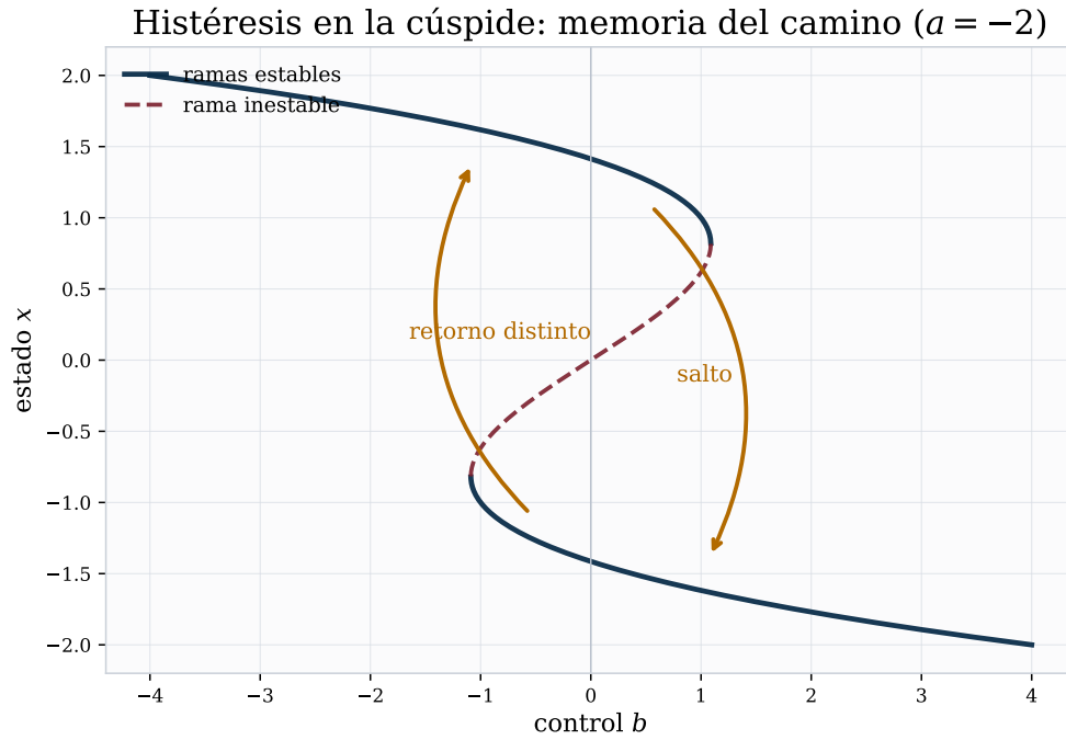
Figura 6: Histéresis en la cúspide para a = -2 . Las ramas sólidas son estables y la rama discontinua es inestable. Los saltos muestran que la trayectoria de ida y la de vuelta no coinciden: una vez institucionalizada una forma de excepción, el retorno de un parámetro no restaura automáticamente el régimen previo.
