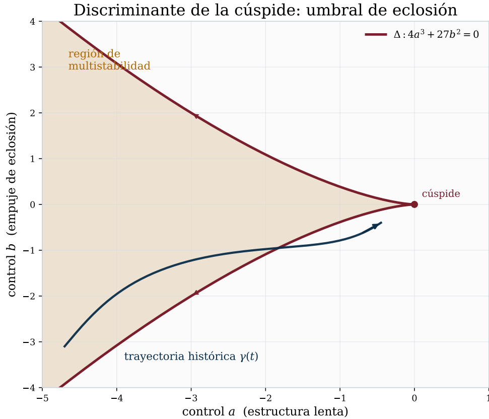
Figura 5: Discriminante de la cúspide en el plano de parámetros (a, b) . La región sombreada indica multistabilidad; la curva roja es \Delta : 4a^3 + 27b^2 = 0 ; la trayectoria azul representa una coyuntura histórica idealizada que se aproxima al umbral de eclosión.
