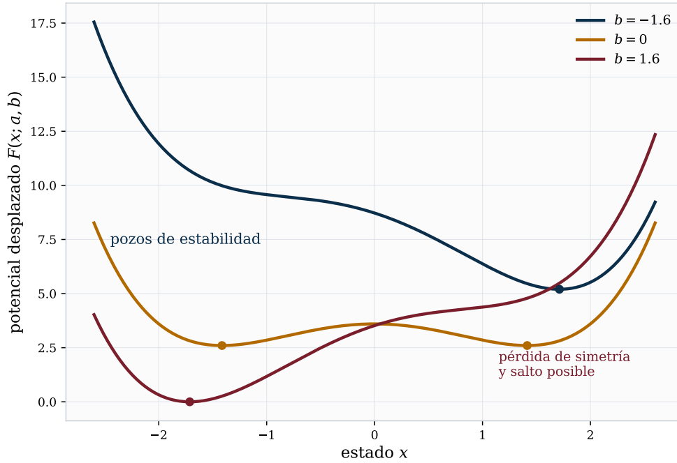
Figura 4: Paisajes de potencial para la cúspide con a = -2 y distintos valores de b . Los pozos representan equilibrios localmente estables; al variar el parámetro de control, la simetría se rompe, una rama se vuelve dominante y el salto deja de parecer accidental. Esta gráfica hace visible la diferencia entre variación continua de parámetros y reorganización cualitativa de la forma.
