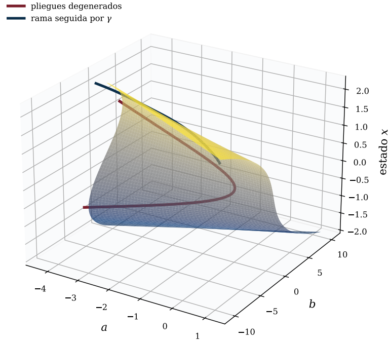
Figura 1: Superficie crítica de la cúspide. La lámina muestra la variedad de equilibrios \Sigma_F para F_x = x^3 + ax + b , las líneas de pliegue donde el Hessiano se degenera y una rama seguida por una trayectoria histórica idealizada. Visualmente, el “huevo” corresponde a una región de estabilidad aparente; la “grieta”, a la aproximación al pliegue; y la “eclosión”, al salto hacia otra rama.
