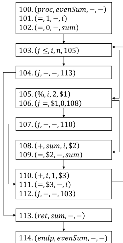
图 8.1 基本块和流图
